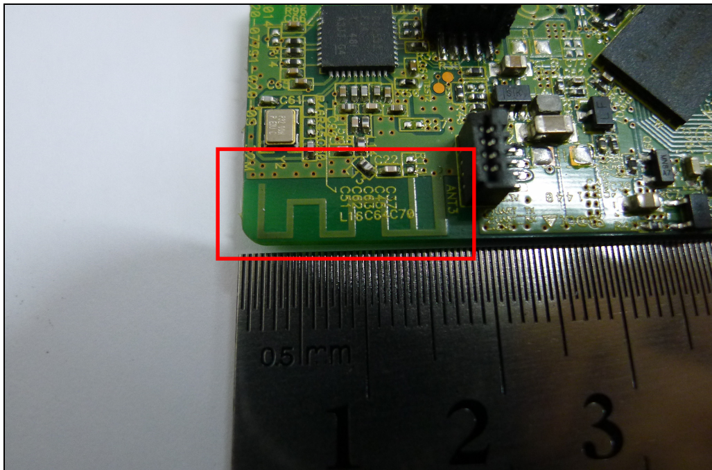
Antenna (Zigbee)
