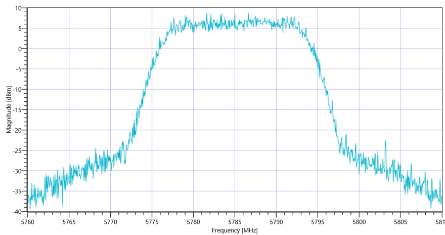
Plot_Common 5Gx-6Gx Peak OP 3MHz-3MHz ~ WLAN5Gx a mode U-NII-3_18082021_093753.png
