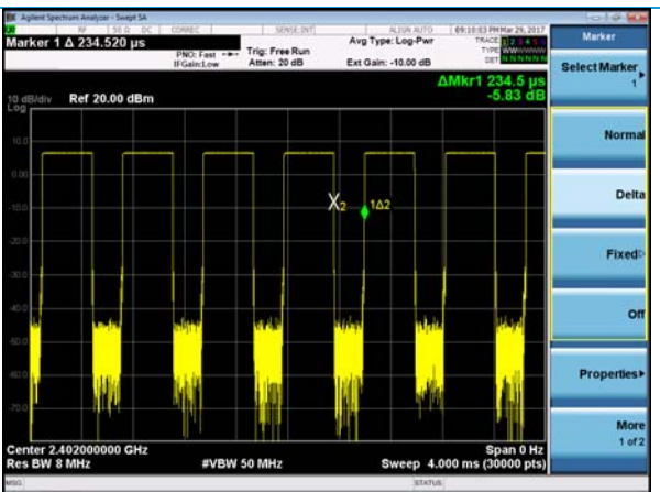
BLE Off-Time
