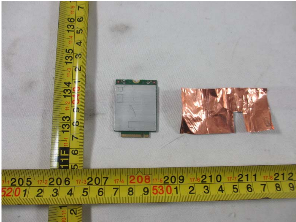
2G-4G module
