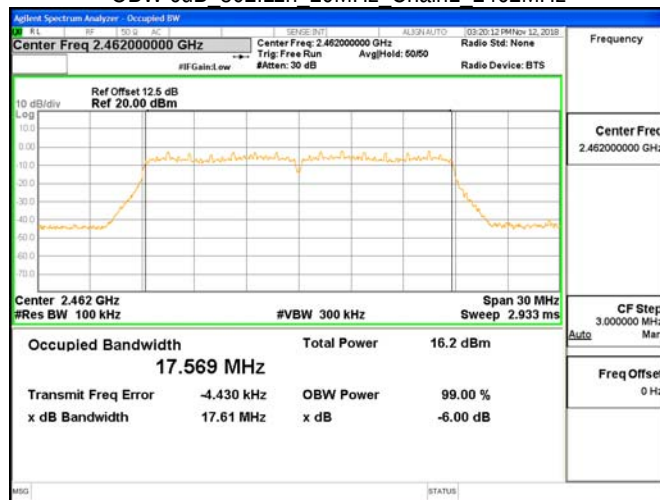
OBW 6dB 802.11n 20MHz Chain1 2462MHz
