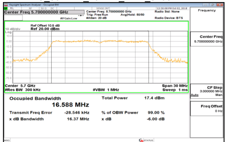
IC 802.11a 20MHz Main 5700MHz
