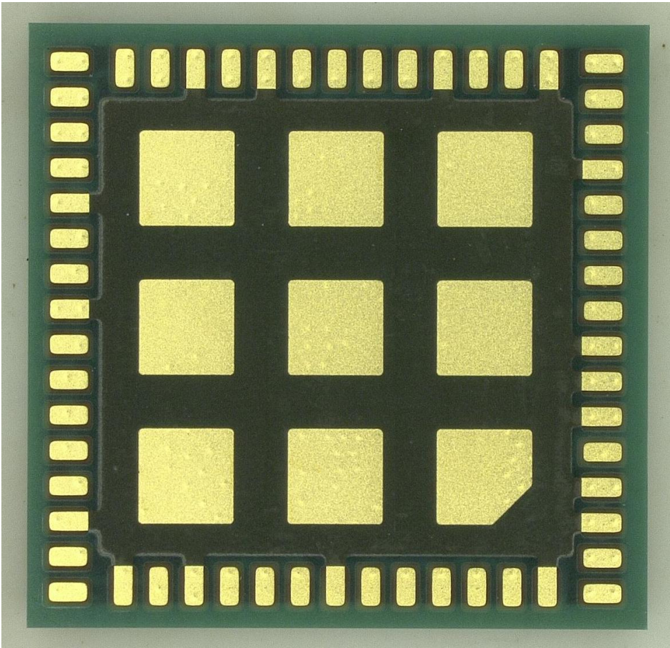
Module(Back)
