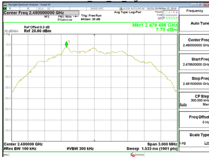
Reference Level BLE 2M HighCH39-2480
