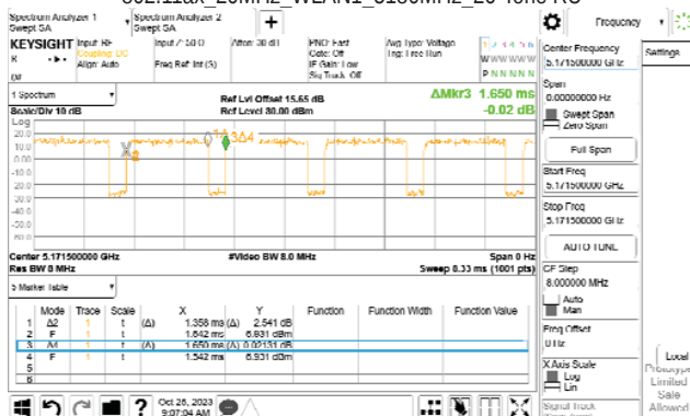
802.11ax 20MHz WLAN1 5180MHz 26-Tone RU
