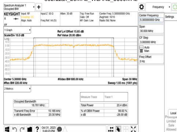
802.11ax_20MHz_WLAN2_5300MHz
