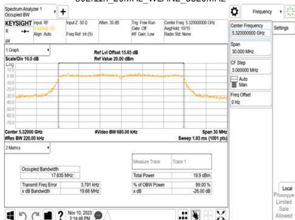
802.11n_20MHz_WLAN2_5320MHz
