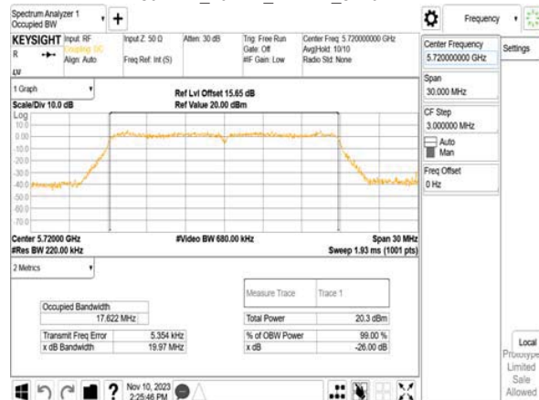
802.11n_20MHz_WLAN1_5720MHz
