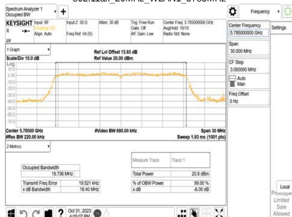
802.11ax_20MHz_WLAN1_5785MHz
