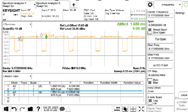
802.11ax_20MHz_WLAN1_5180MHz_106-Tone RU
