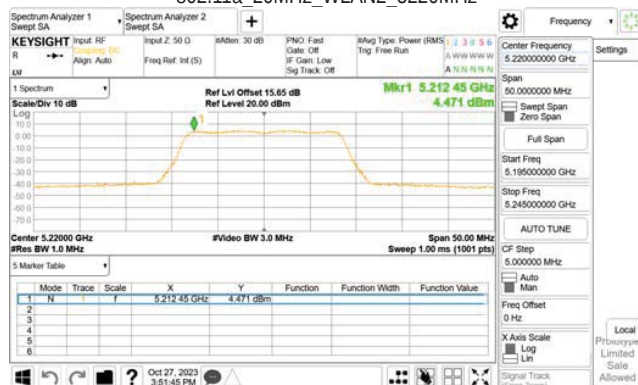
802.11a_20MHz_WLAN2_5220MHz
