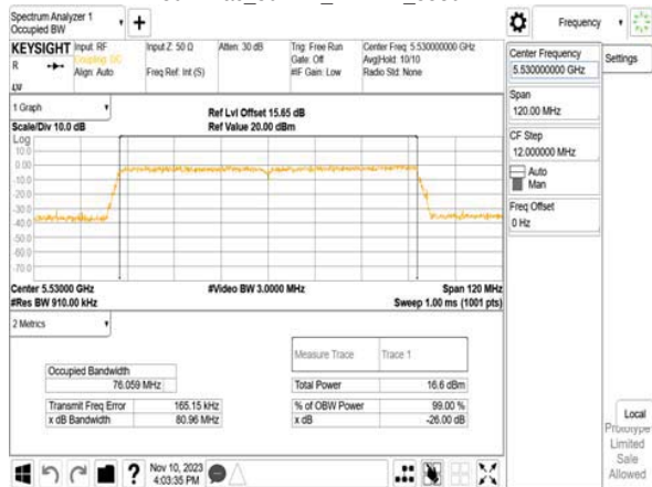
802.11ac_80MHz_WLAN1_5530MHz
