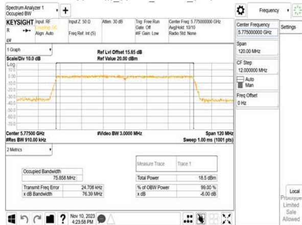
802.11ac_80MHz_WLAN1_5775MHz
