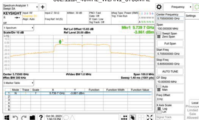
802.11ax_40MHz_WLAN1_5755MHz_RU242_61
