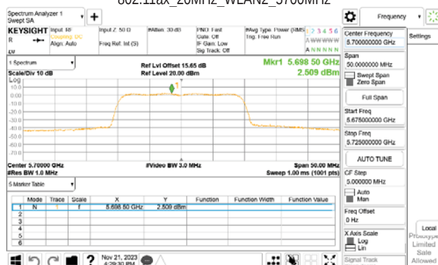
802.11ax_20MHz_WLAN2_5700MHz_RU26_8
