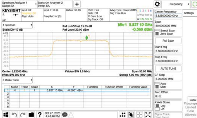
802.11ax_20MHz_WLAN2_5825MHz_RU26 8
