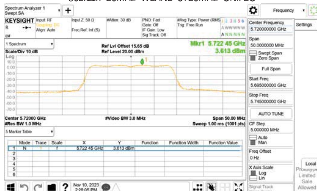
802.11n_20MHz_WLAN2_5720MHz_UNII 2C
