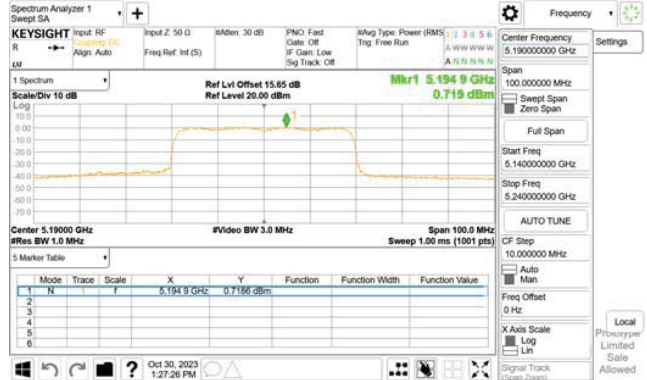
802.11ax_40MHz_WLAN1_5190MHz_RU242 61
