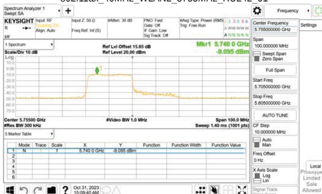
802.11ax_40MHz_WLAN2_5755MHz_RU242 61
