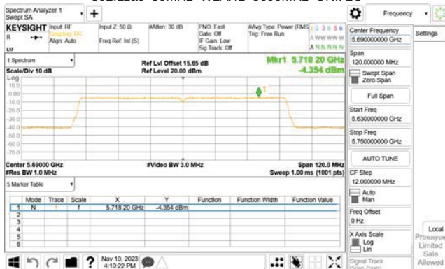
802.11ac_80MHz_WLAN1_5690MHz_UNII 3
