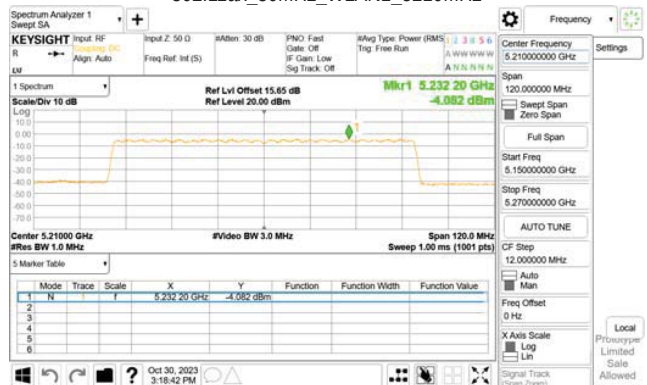
802.11ax_80MHz_WLAN1_5210MHz_RU484 65
