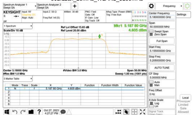
802.11ax_20MHz_WLAN1_5180MHz_RU26_0
