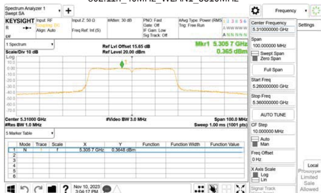
802.11n_40MHz_WLAN1_5310MHz
