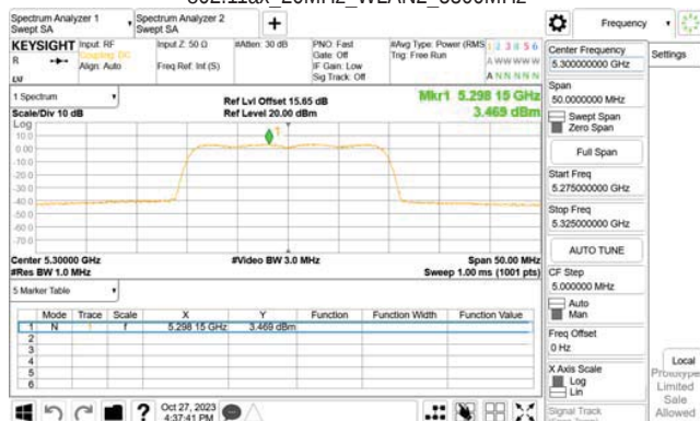
802.11ax_20MHz_WLAN2_5300MHz
