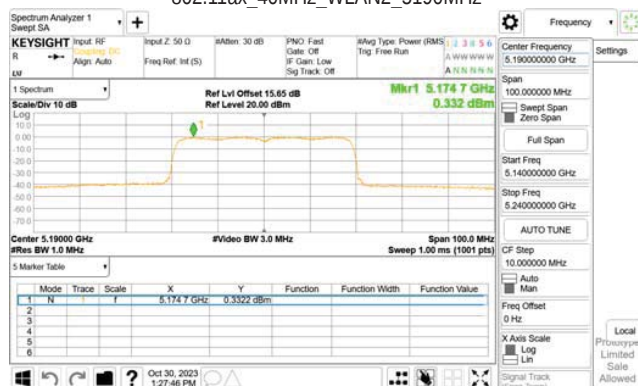
802.11ax_40MHz_WLAN2_5190MHz_RU242_61
