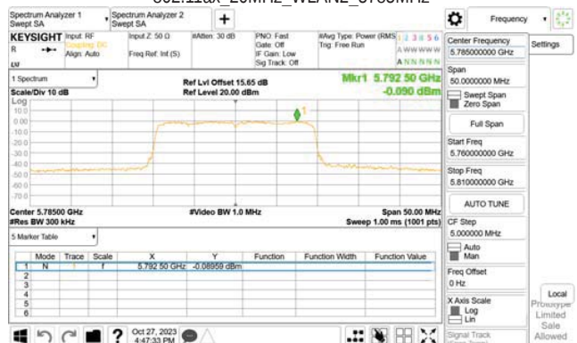
802.11ax_20MHz_WLAN2_5785MHz
