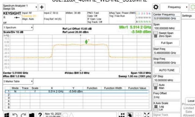
802.11ax_40MHz_WLAN2_5510MHz
