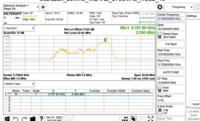
802.11ax_20MHz_WLAN2_5700MHz_RU52_40
