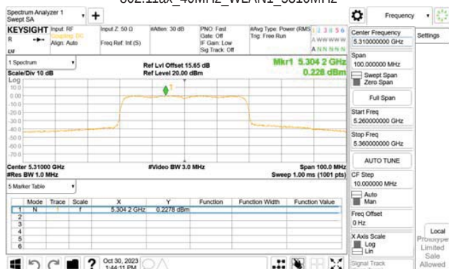
802.11ax_40MHz_WLAN1_5310MHz_RU242_62
