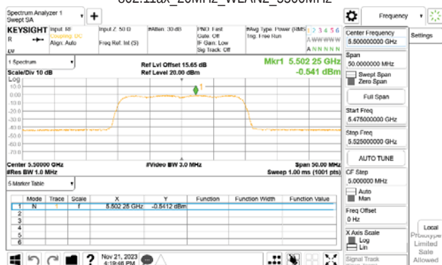
802.11ax_20MHz_WLAN2_5500MHz_RU26_0
