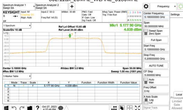
802.11ax_20MHz_WLAN2_5180MHz_RU26_0
