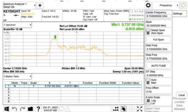
802.11ax_20MHz_WLAN2_5745MHz_RU52_37
