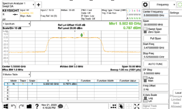
802.11ax_20MHz_WLAN1_5500MHz_RU26_0
