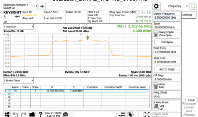
802.11ax_20MHz_WLAN1_5700MHz_RU26_8
