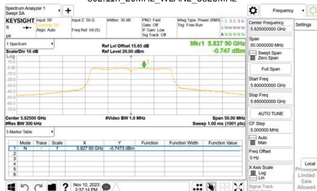
802.11n_20MHz_WLAN2_5825MHz
