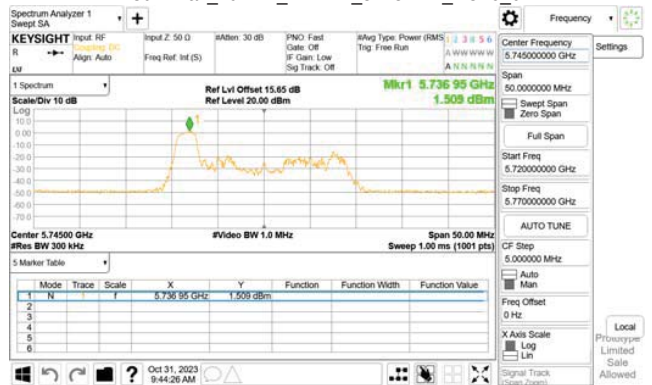
802.11ax_20MHz_WLAN1_5745MHz_RU52_37
