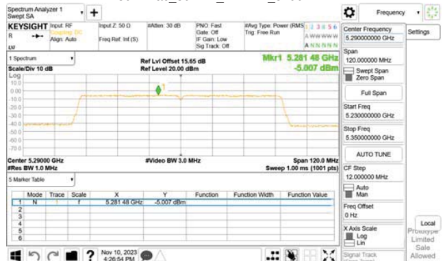
802.11ac_80MHz_WLAN1_5290MHz
