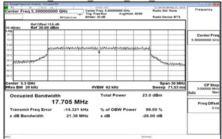
FCC 802.11n 20MHz_CH0_5300MHz
