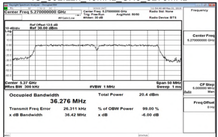
IC 802.11n 40MHz CH0 5270MHz
