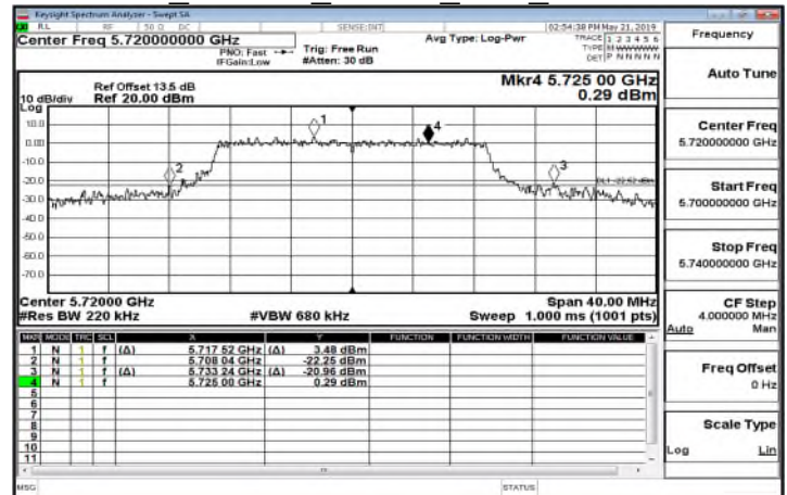
FCC 802.11n 20MHz CH1 5720MHz
