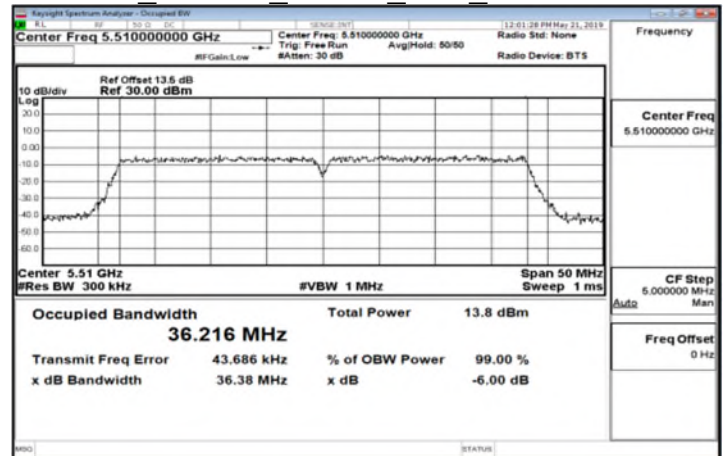
IC 802.11n 40MHz CH1 5510MHz
