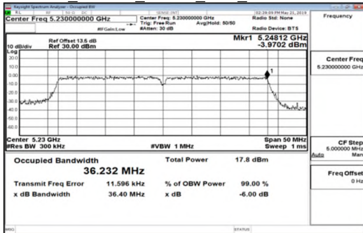
IC 802.11n 40MHz CH1 5230MHz
