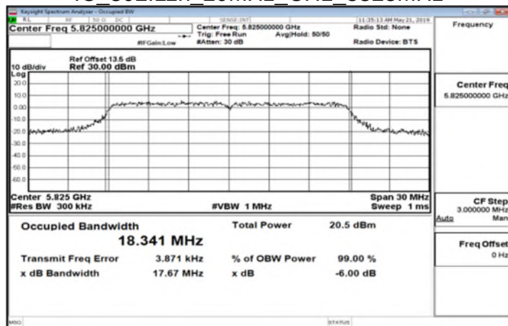
IC 802.11n 20MHz CH1 5825MHz
