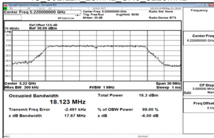
IC 802.11n 20MHz CH0 5220MHz
