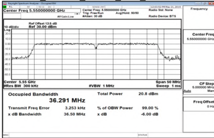
IC 802.11n 40MHz CH0 5550MHz
