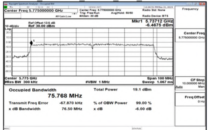
IC 802.11ac 80MHz_CH0 5775MHz
