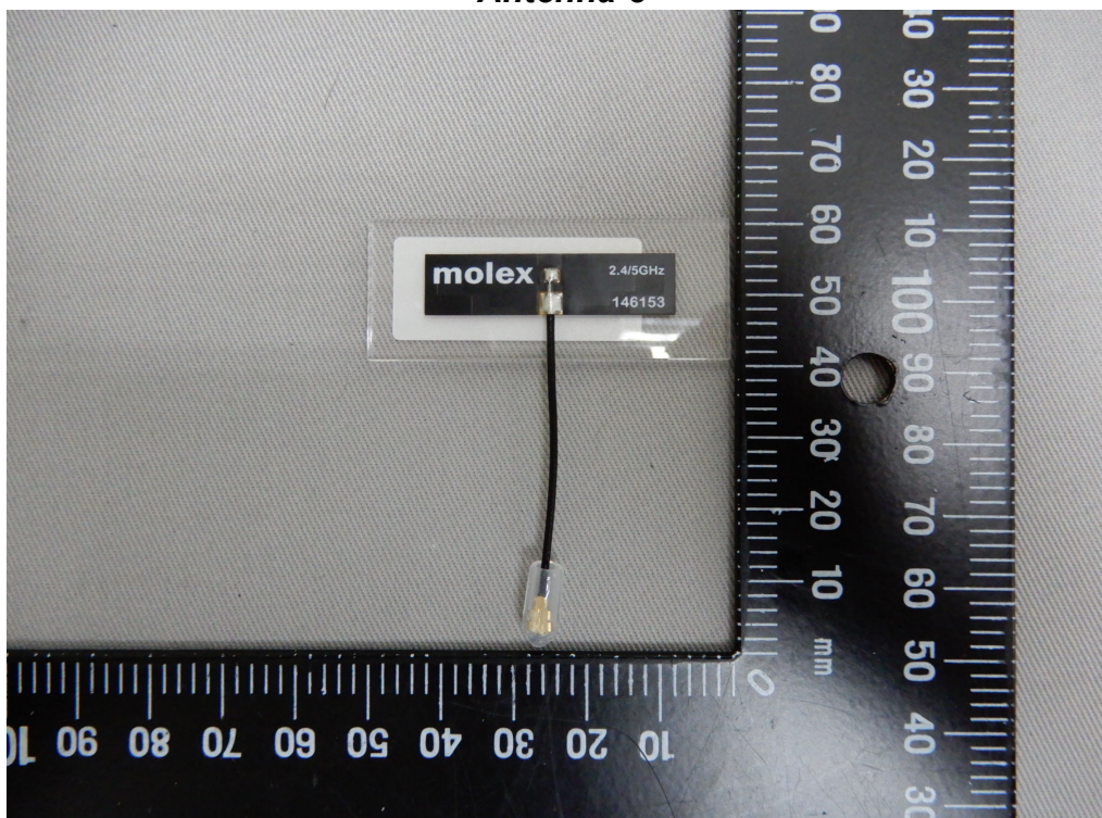
Antenna-3
