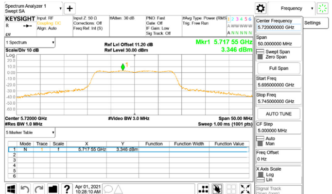
PSD_802.11a_20MHz_Chain0_5720MHz_UNII 3
