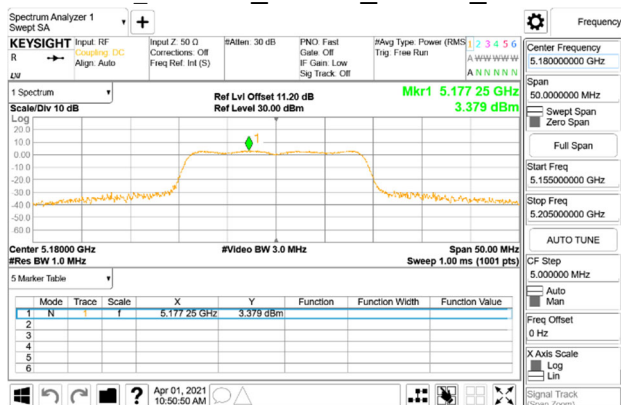
PSD_802.11n_20MHz_Chain0_5180MHz
