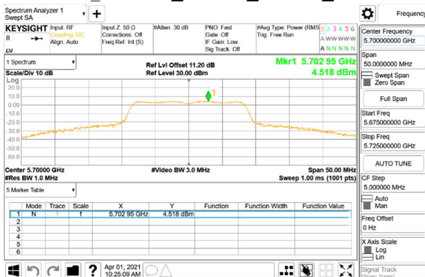
PSD_802.11a_20MHz_Chain0_5700MHz
