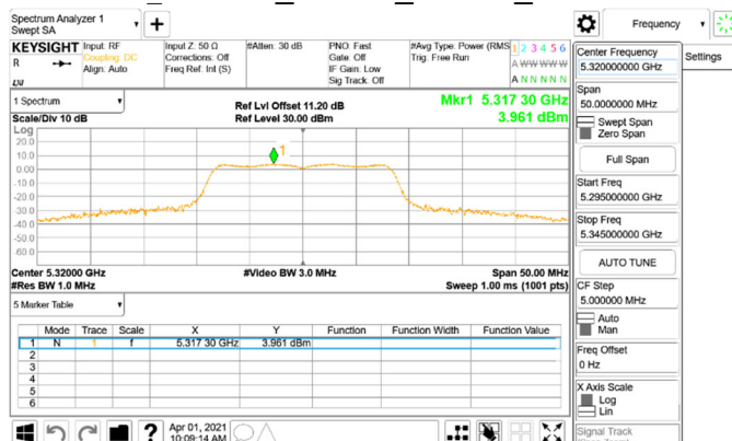
PSD_802.11a_20MHz_Chain0_5320MHz
