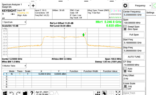
PSD_802.11n_40MHz_Chain0_5230MHz
