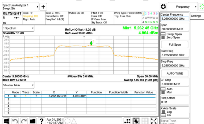
PSD_802.11n_20MHz_Chain0_5260MHz
