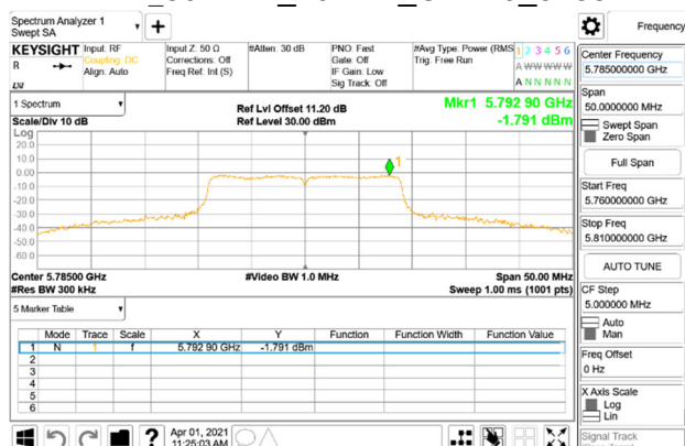
PSD_802.11n_20MHz_Chain0_5785MHz
