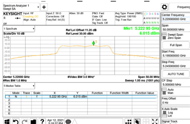
PSD_802.11a_20MHz_Chain0_5220MHz
