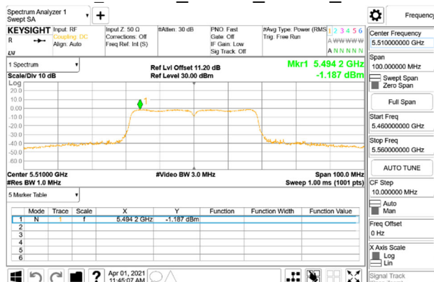
PSD_802.11n_40MHz_Chain0_5510MHz
