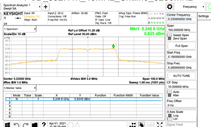
PSD 802.11n_40MHz_Chain0_5230MHz
