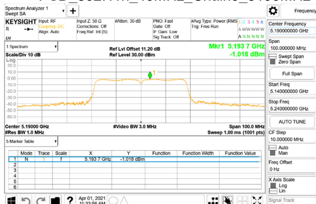
PSD 802.11n_40MHz_Chain0_5190MHz
