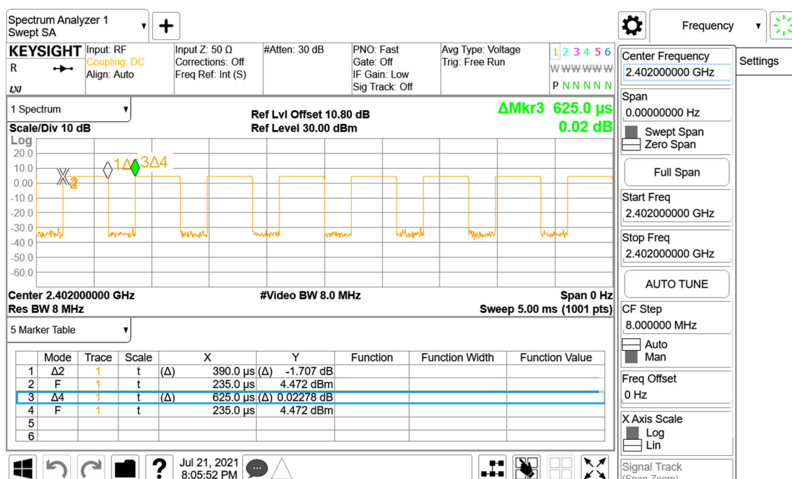
Duty Cycle BLE 1M LowCH00-2402
