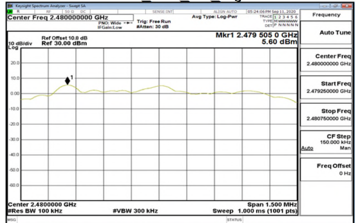
Reference Level BLE 2M HighCH39-2480
