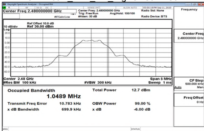
OBW 6dB BLE 1M HighCH39-2480
