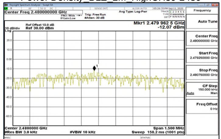
Power Density BLE 2M HighCH39-2480
