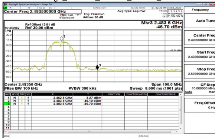
Band Edge_802.11b_20MHz_Chain0_2462MHz
