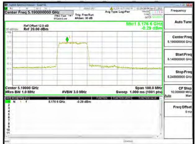
802.11ax_40MHz_Chain0_5190MHz_RU242_61
