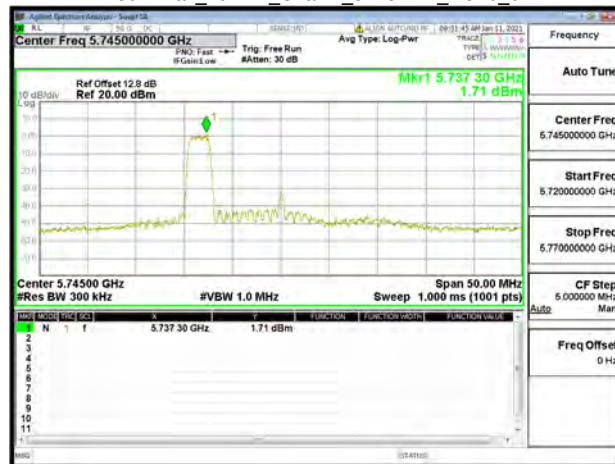
802.11ax_20MHz_Chain1_5745MHz_RU52_37
