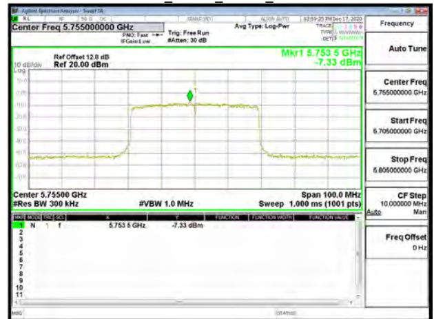
802.11ax_40MHz_Chain1_5755MHz_RU242_61
