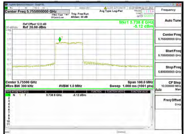
802.11ax_40MHz_Chain1_5755MHz_RU242_61
