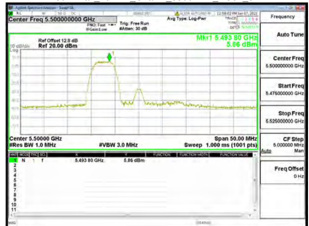
802.11ax_20MHz_Chain1_5500MHz_RU52_37
