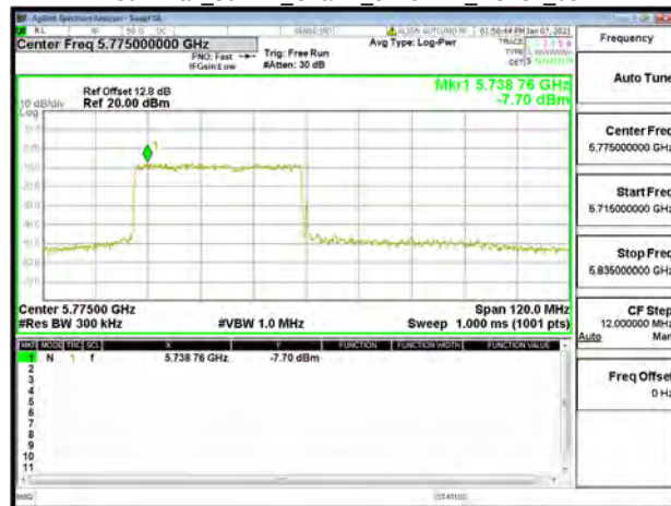
802.11ax_80MHz_Chain1_5775MHz_RU484_66
