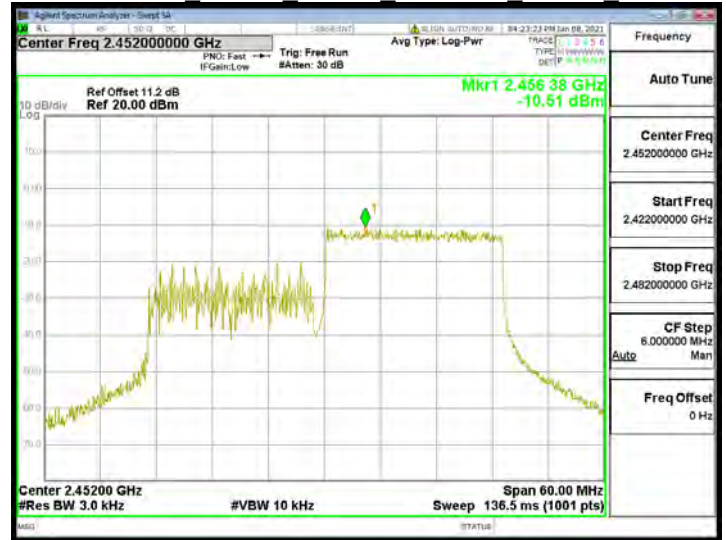
802.11ax 40MHz Chain1 2452MHz RU242 62
