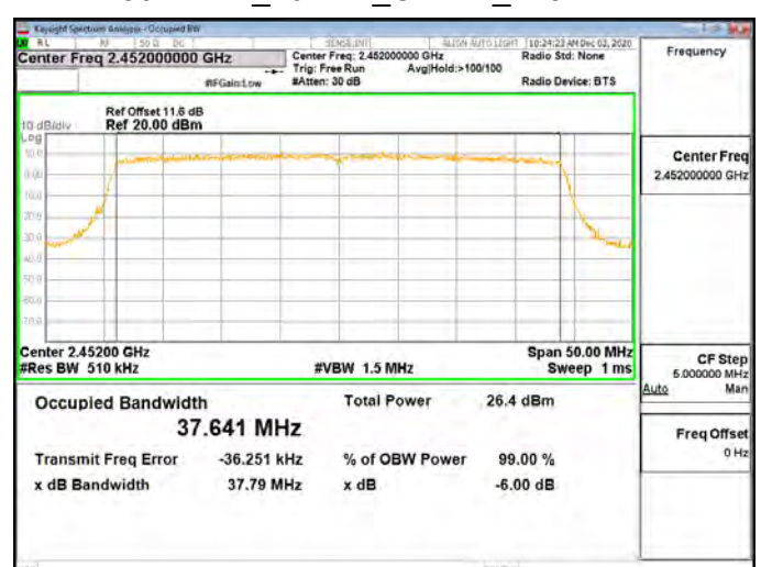
802.11ax 40MHz Chain1 2452MHz
