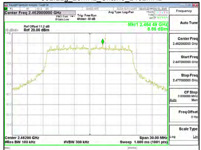
802.11g 20MHz Chain0 2462MHz
