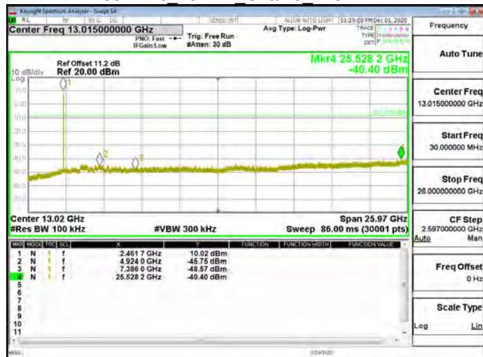
802.11b 20MHz Chain0 2462MHz
