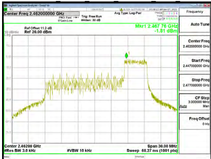
802.11ax 20MHz Chain0 2462MHz RU106 54
