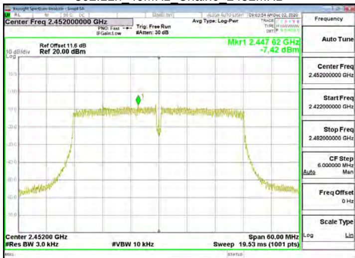
802.11n 40MHz Chain0 2452MHz
