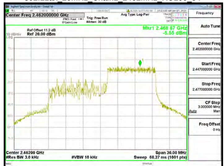
802.11ax 20MHz Chain1 2462MHz RU106 54
