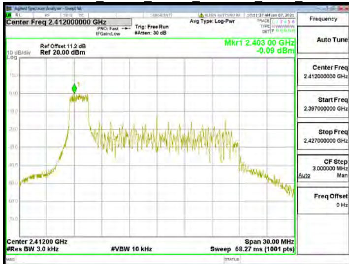
802.11ax 20MHz Chain0 2412MHz RU52 37
