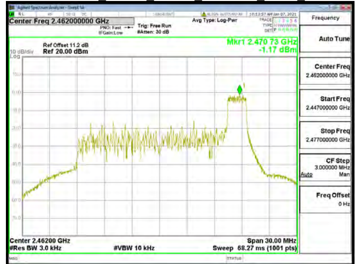
802.11ax 20MHz Chain1 2462MHz RU52 40
