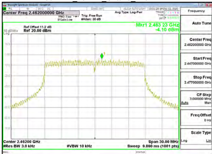
802.11n 20MHz Chain0 2462MHz
