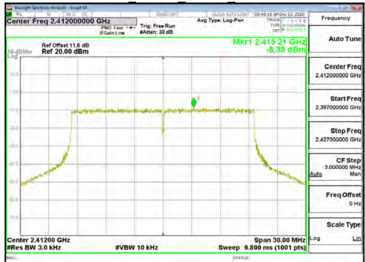
802.11ax 20MHz Chain1 2412MHz RU26 0
