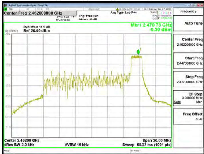
802.11ax 20MHz Chain0 2462MHz RU52 40
