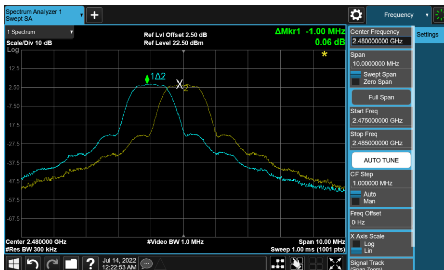
Mode2/CH78/2480MHz
