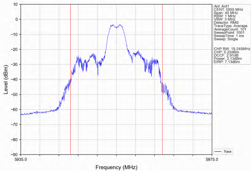
802.11ax(HE20)_LCH_5955MHz_RU26_Right_Ant1_NTNV
