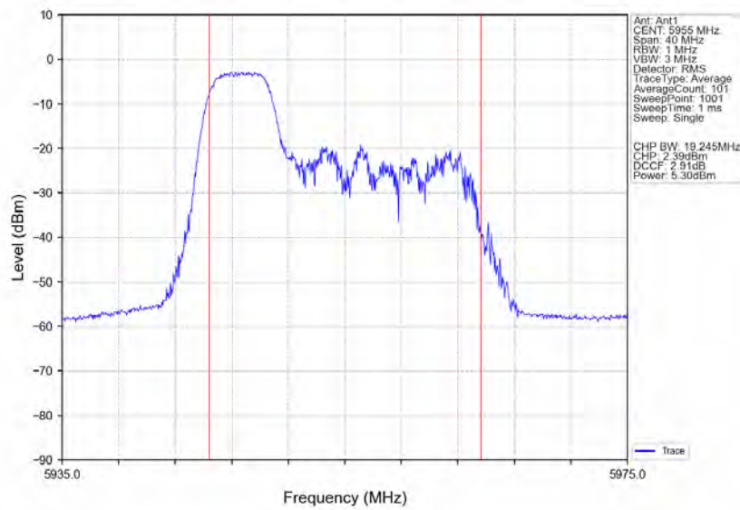
802.11ax(HE20)_LCH_5955MHz_RU52_Right_Ant1_NTNV
