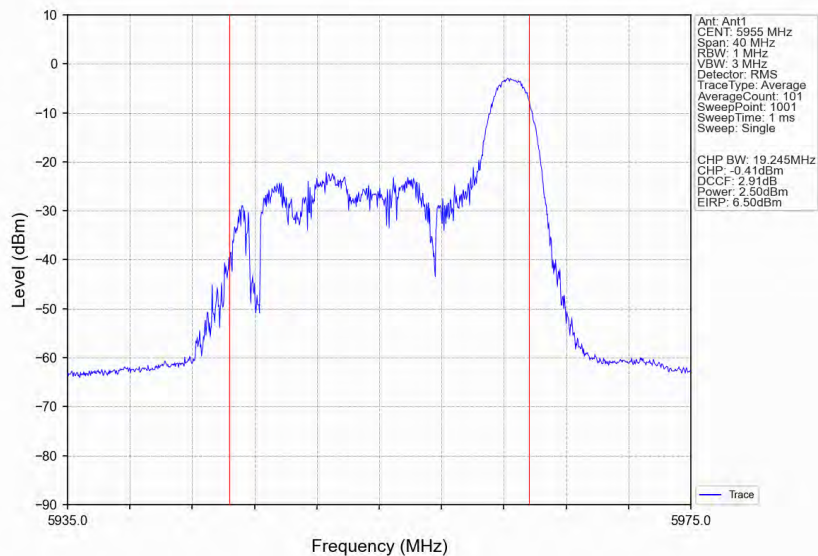
802.11ax(HE20)_LCH_5955MHz_RU26_Right_Ant1_NTNV
