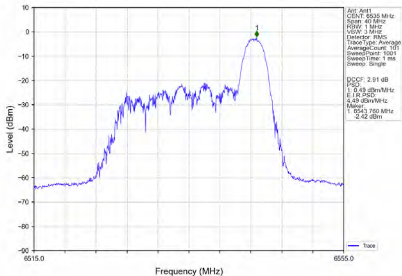
802.11ax(HE20)_LCH_6535MHz_RU26_Right_Ant1_NTNV
