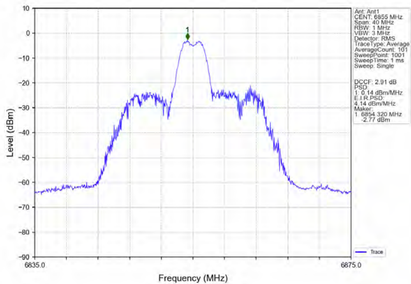
802.11ax(HE20) HCH_6855MHz_RU26_Right_Ant1_NTNV
