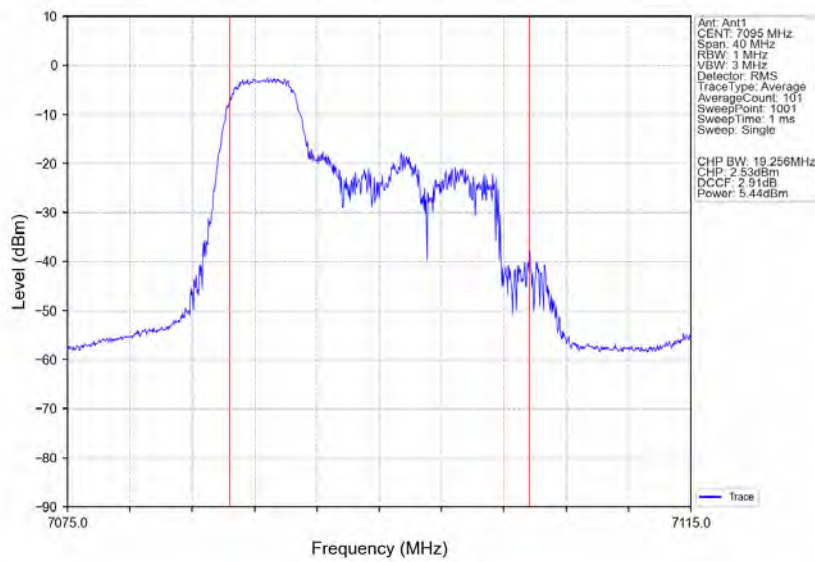
802.11ax(HE20) HCH_7095MHz_RU52_Right_Ant1_NTNV
