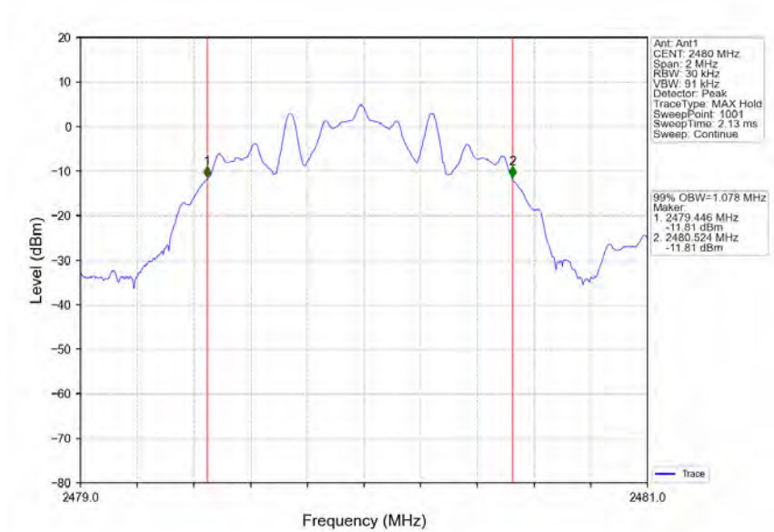
S8_HCH_2480MHz_Ant1_NTNV
