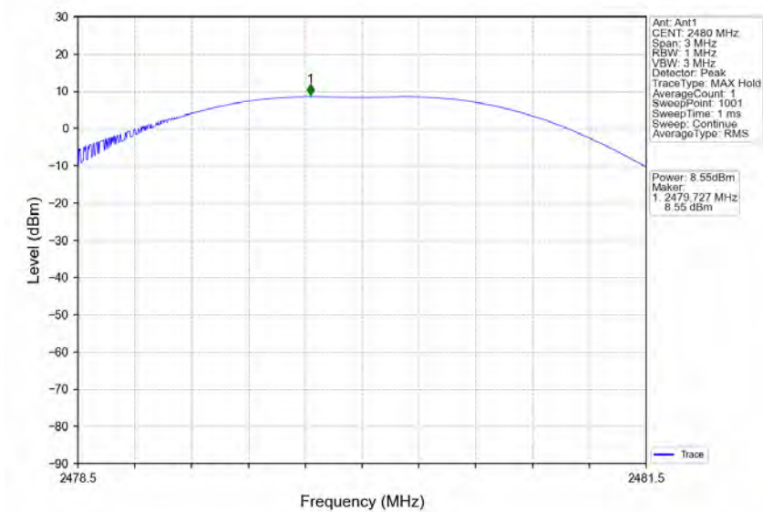
S2_HCH_2480MHz_Ant1_NTNV
