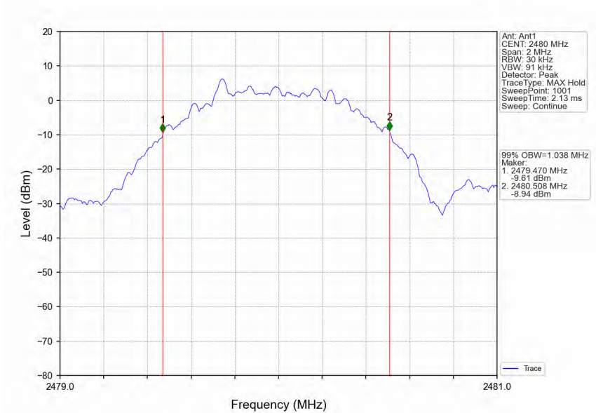
S2_HCH_2480MHz_Ant1_NTNV
