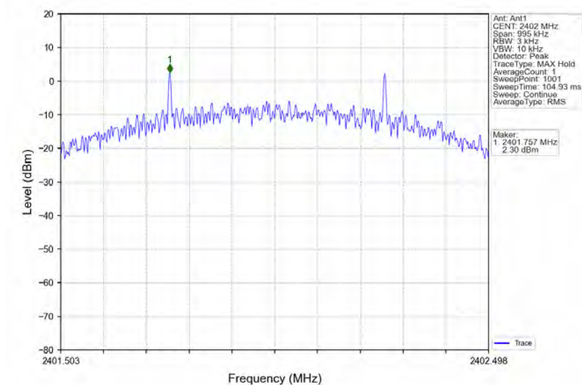
S2_LCH_2402MHz_Ant1_NTNV
