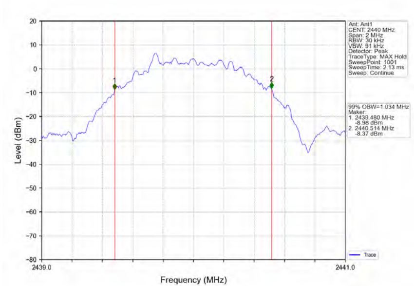
S2_MCH_2440MHz_Ant1_NTNV
