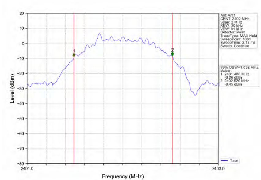
S2_LCH_2402MHz_Ant1_NTNV
