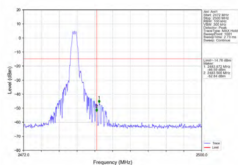
S8_HCH_2480MHz_Ant1_NTNV
