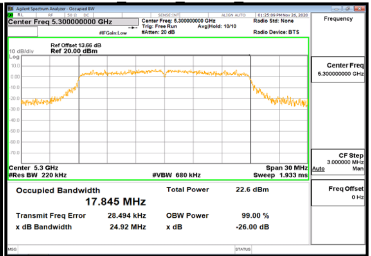
802.11n_20MHz_Chain0_5300MHz
