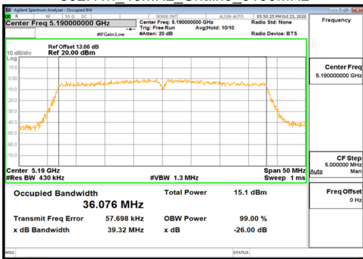
802.11n 40MHz Chain0 5190MHz
