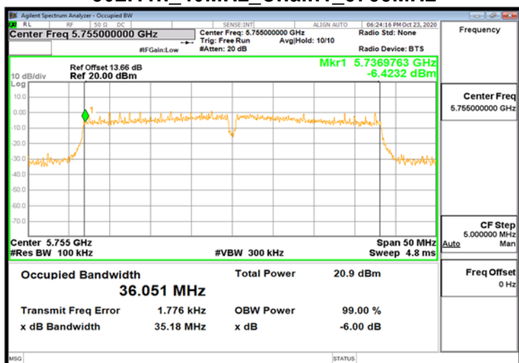
802.11n_40MHz_Chain1_5755MHz
