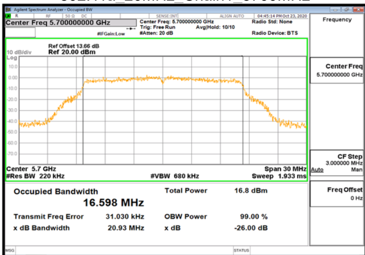
802.11a 20MHz Chain1_5700MHz
