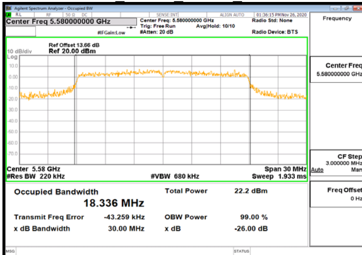
802.11n 20MHz Chain0 5580MHz
