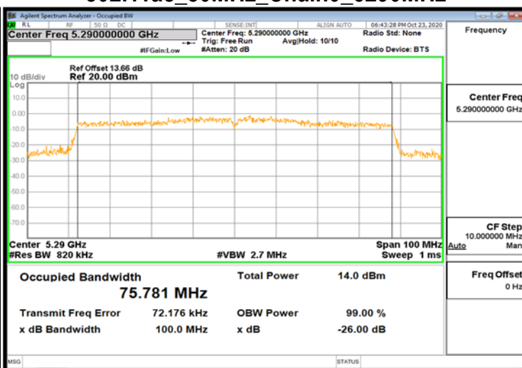
802.11ac_80MHz_Chain0_5290MHz
