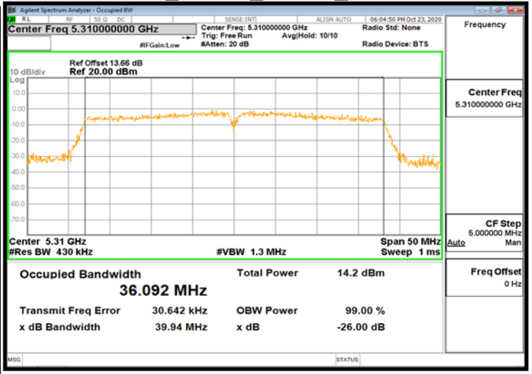
802.11n 40MHz Chain0 5310MHz
