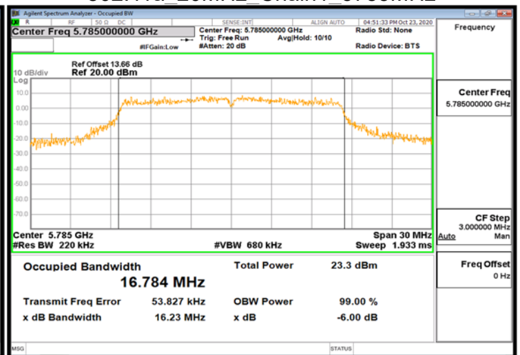
802.11a 20MHz Chain1_5785MHz
