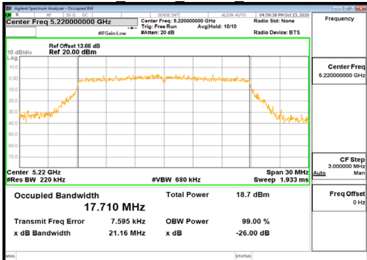
802.11n 20MHz Chain1 5220MHz
