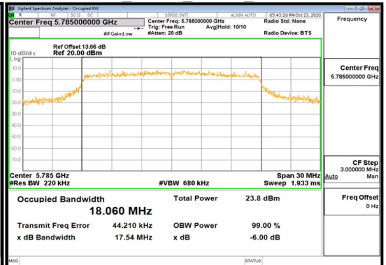
802.11n 20MHz Chain0 5785MHz
