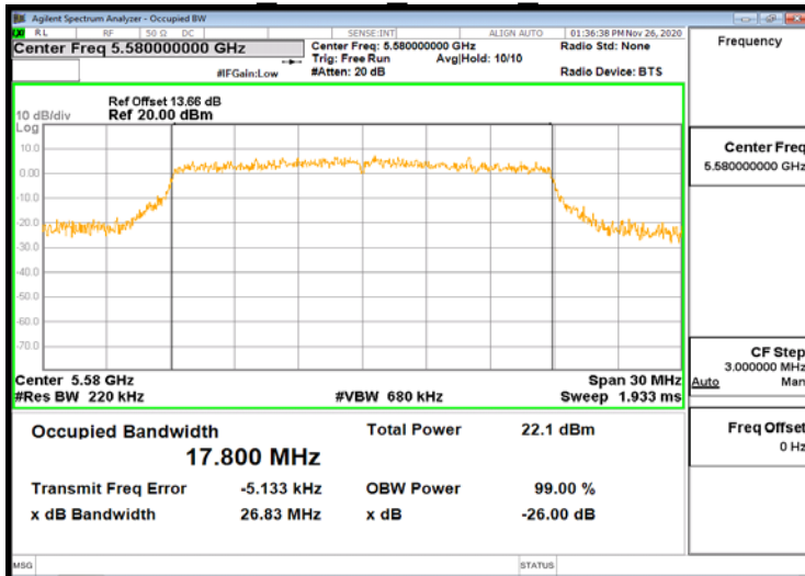
802.11n 20MHz Chain1 5580MHz
