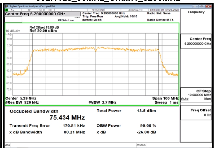
802.11ac_80MHz_Chain1_5290MHz
