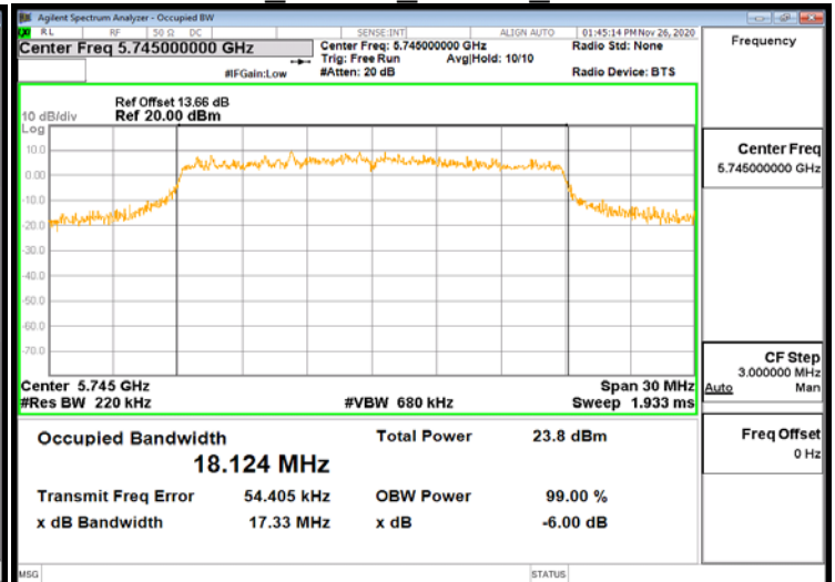
802.11n 20MHz Chain1 5745MHz
