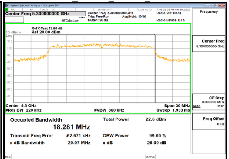
802.11n 20MHz Chain1 5300MHz
