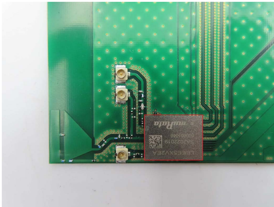
RF Module
