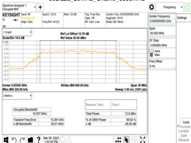
802.11a_20MHz_Chain0_6855MHz
