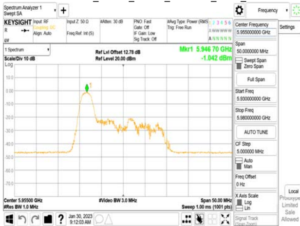
802.11ax_20MHz_Chain0_5955MHz_RU52_37
