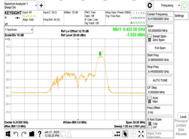
802.11ax_20MHz_Chain0_6415MHz_RU52_40
