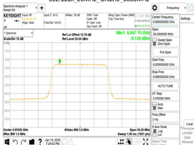
802.11ax_20MHz_Chain0_6855MHz
