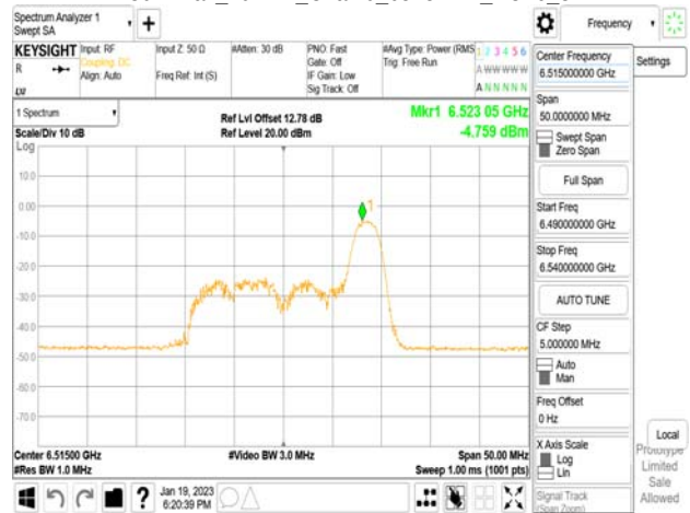
802.11ax_20MHz_Chain0_6515MHz_RU52_40
