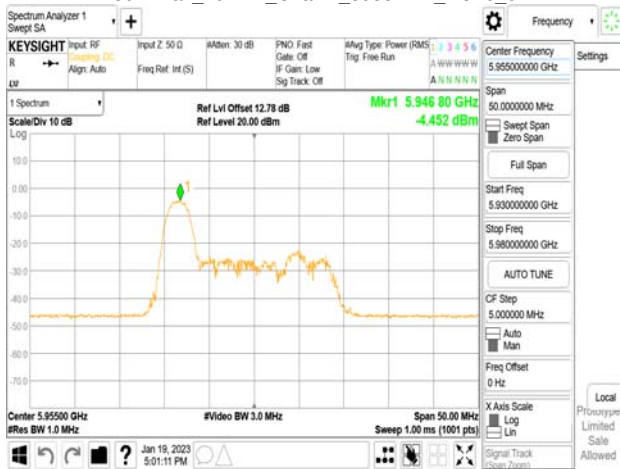
802.11ax_20MHz_Chain1_5955MHz_RU52_37
