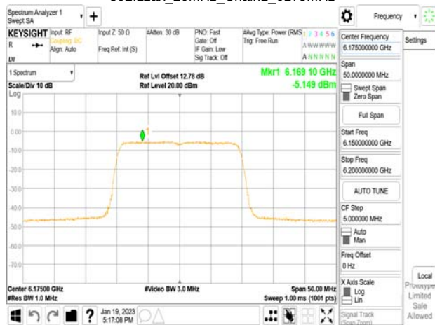
802.11ax_20MHz_Chain1_6175MHz
