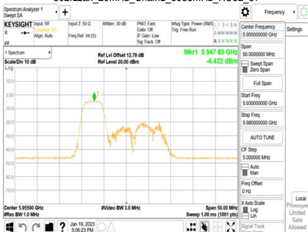
802.11ax_20MHz_Chain1_5955MHz_RU106_53
