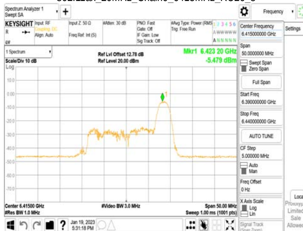
802.11ax_20MHz_Chain0_6415MHz_RU52_40
