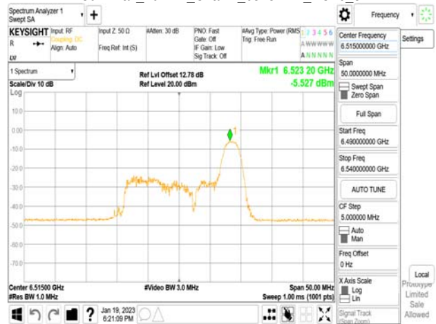
802.11ax_20MHz_Chain1_6515MHz_RU52_40
