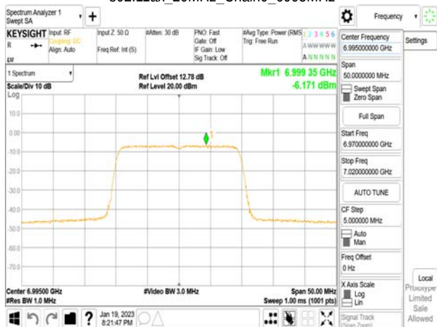
802.11ax_20MHz_Chain0_6995MHz
