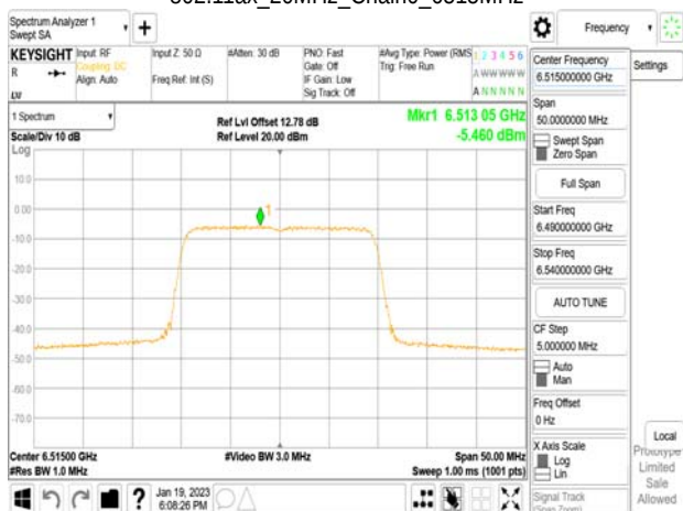
802.11ax_20MHz_Chain0_6515MHz
