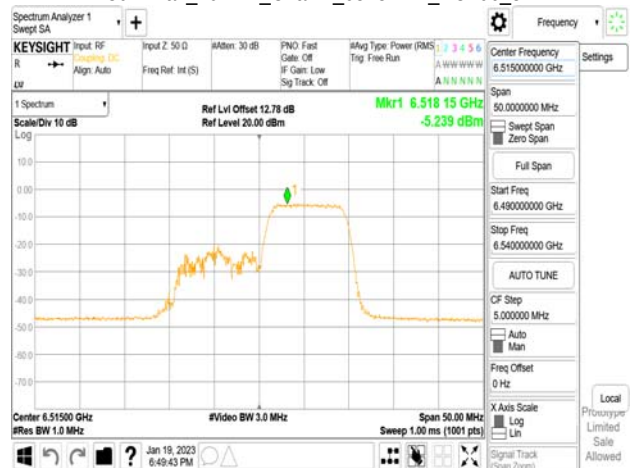
802.11ax_20MHz_Chain1_6515MHz_RU106_54
