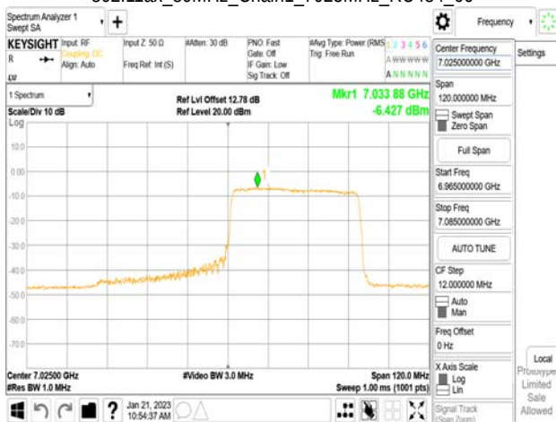
802.11ax_80MHz_Chain1_7025MHz_RU484_66
