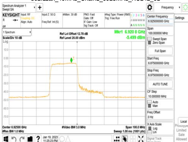
802.11ax_40MHz_Chain1_6925MHz_RU242_61
