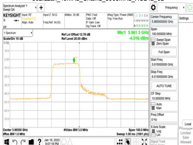
802.11ax_40MHz_Chain1_5965MHz_RU242_61
