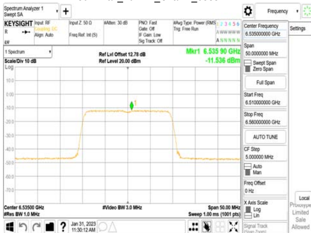
802.11ax_20MHz_Chain1_6535MHz_RU26_0
