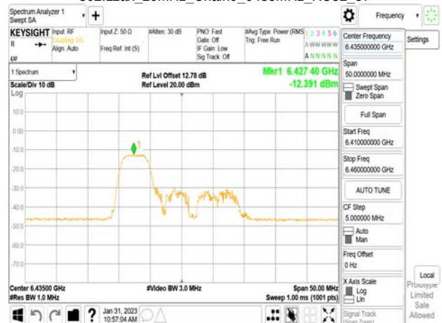
802.11ax_20MHz_Chain0_6435MHz_RU52_37
