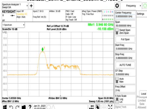
802.11ax_20MHz_Chain1_5955MHz_RU26_0
