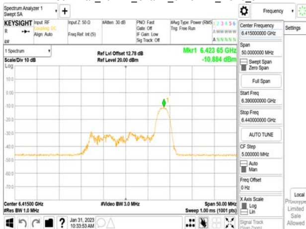
802.11ax_20MHz_Chain1_6415MHz_RU52_40
