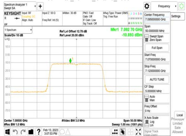
802.11ax_20MHz_Chain0_7095MHz_RU26_8
