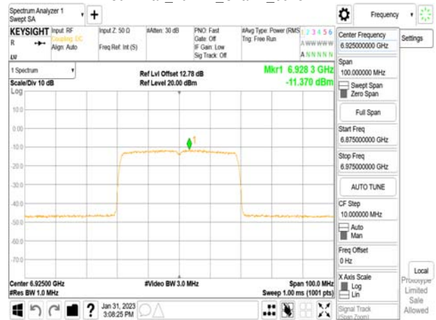
802.11ax_40MHz_Chain1_6925MHz_RU242_61
