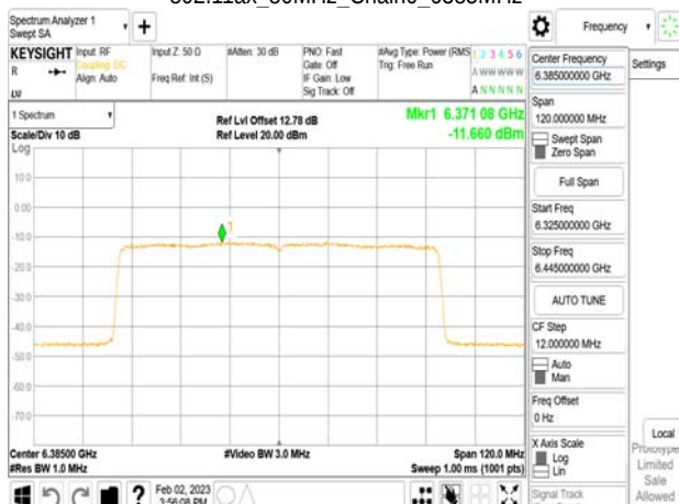
802.11ax_80MHz_Chain0_6385MHz
