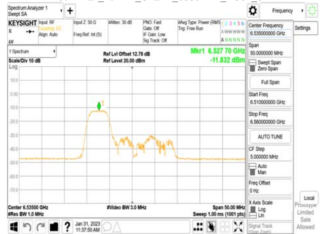
802.11ax_20MHz_Chain1_6535MHz_RU106_53
