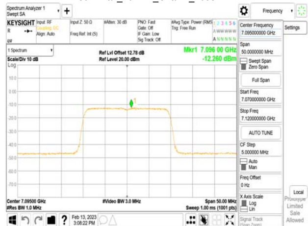
802.11ax_20MHz_Chain1_7095MHz_RU26_8
