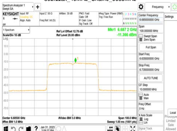
802.11ax_40MHz_Chain0_6685MHz
