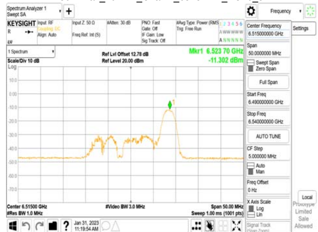
802.11ax_20MHz_Chain1_6515MHz_RU52_40
