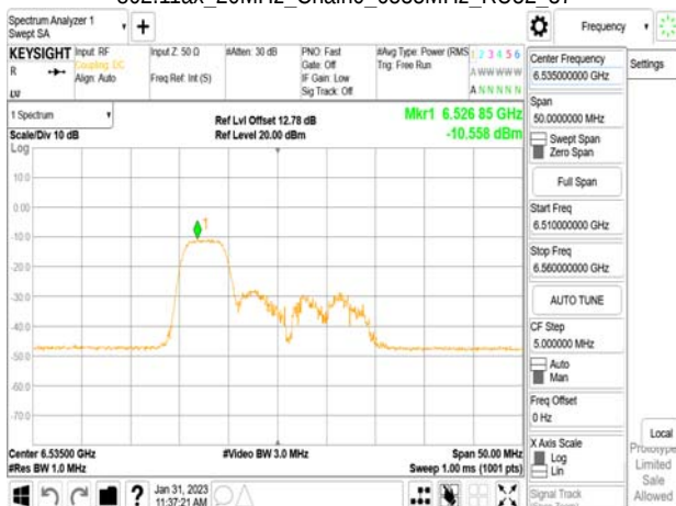
802.11ax_20MHz_Chain0_6535MHz_RU52_37
