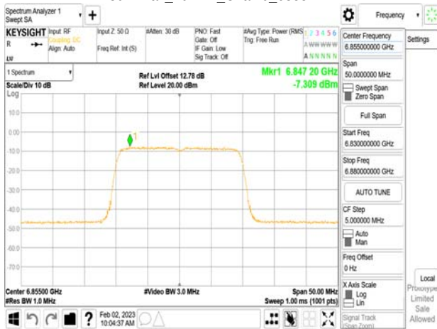
802.11ax_20MHz_Chain0_6855MHz_RU26_8
