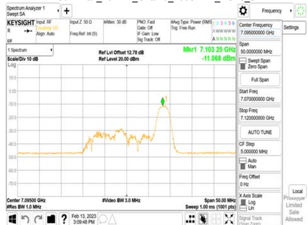
802.11ax_20MHz_Chain0_7095MHz_RU52_40
