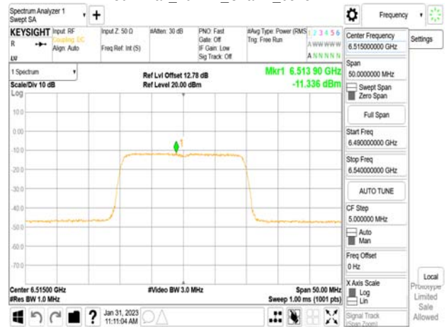
802.11ax_20MHz_Chain1_6515MHz_RU26_8
