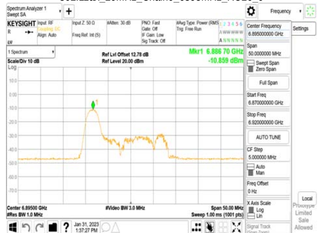
802.11ax_20MHz_Chain0_6895MHz_RU26_0
