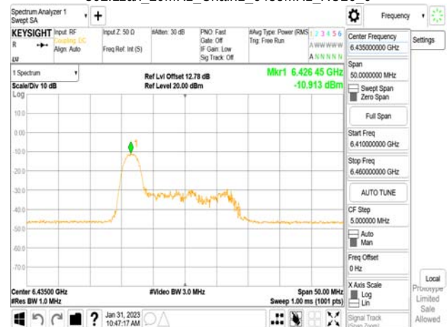
802.11ax_20MHz_Chain1_6435MHz_RU26_0
