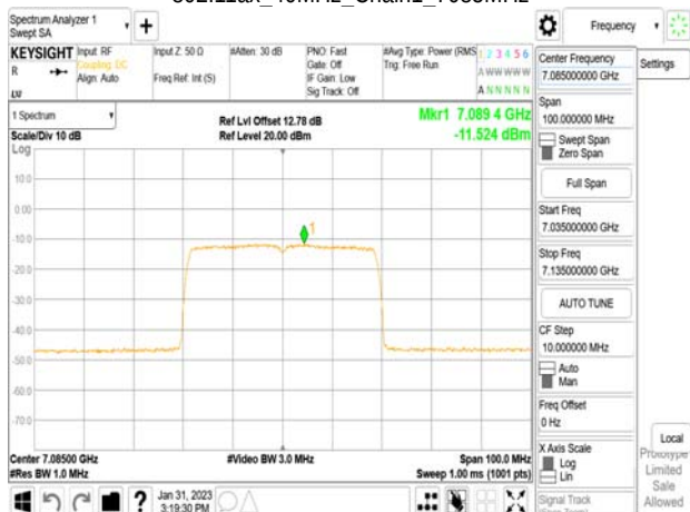
802.11ax_40MHz_Chain1_7085MHz_RU242_62
