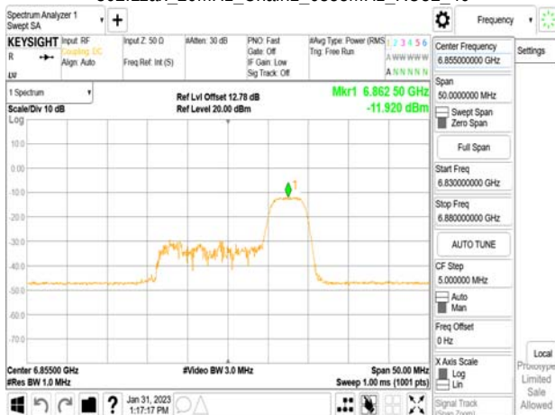
802.11ax_20MHz_Chain1_6855MHz_RU52_40
