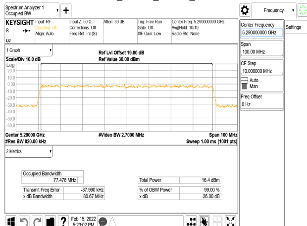
802.11ax_80MHz_Chain0_5290MHz
