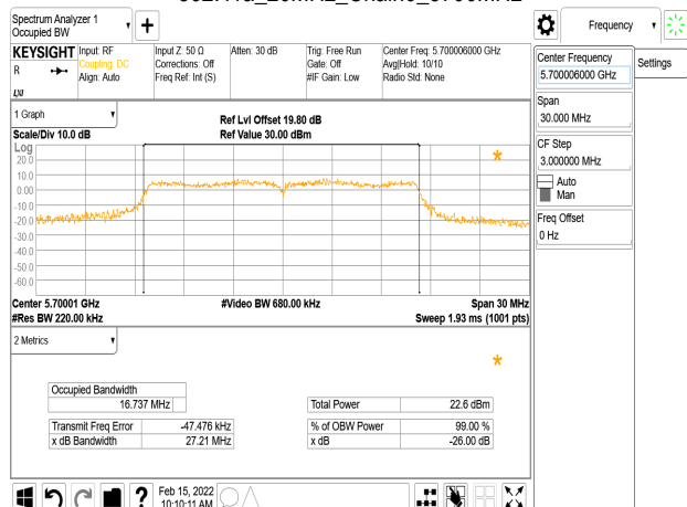
802.11a_20MHz_Chain0_5700MHz
