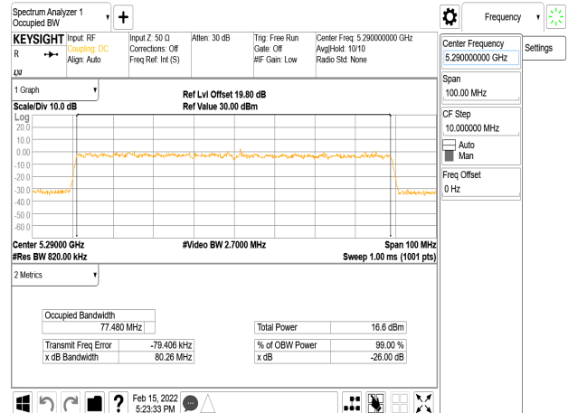
802.11ax_80MHz_Chain1_5290MHz
