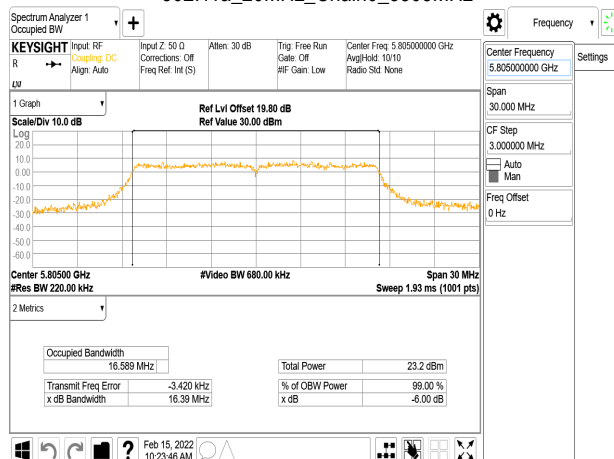
802.11a_20MHz_Chain0_5805MHz
