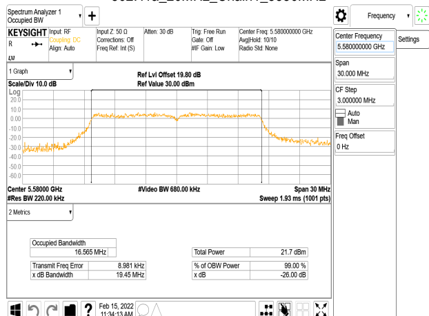
802.11a_20MHz_Chain1_5580MHz
