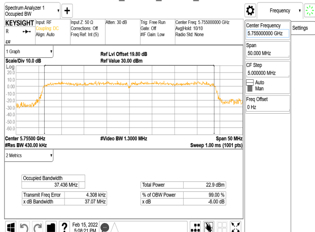
802.11ax_40MHz_Chain0_5755MHz
