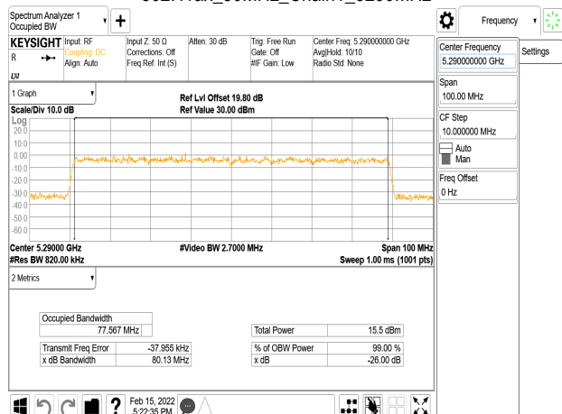
802.11ax_80MHz_Chain1_5290MHz
