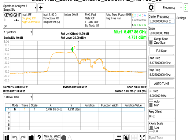
802.11ax_20MHz_Chain0_5500MHz_RU26_0
