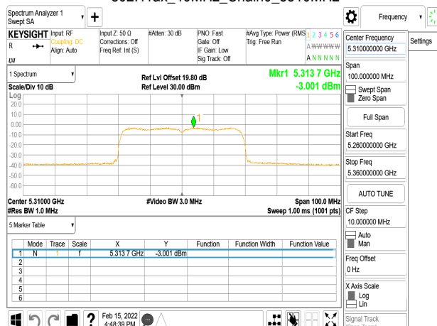
802.11ax_40MHz_Chain0_5310MHz_RU242_62
