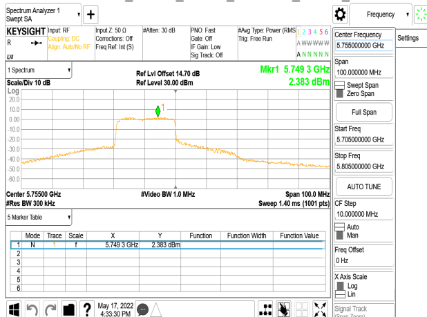
802.11ax_40MHz_Chain0_5755MHz_RU242_61
