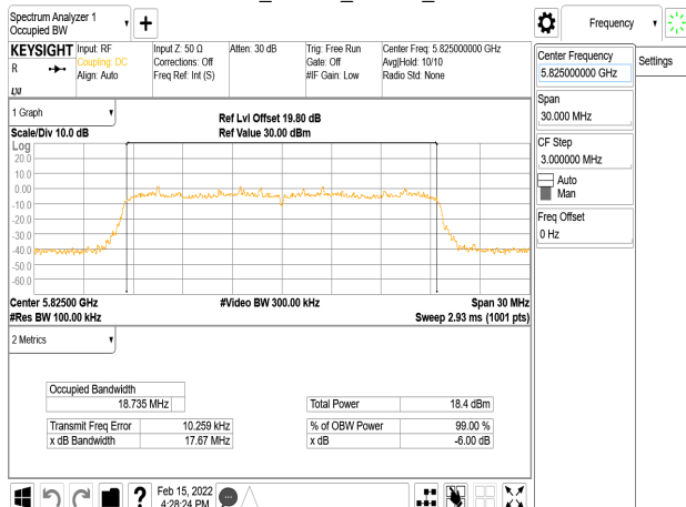
802.11ax_20MHz_Chain1_5825MHz
