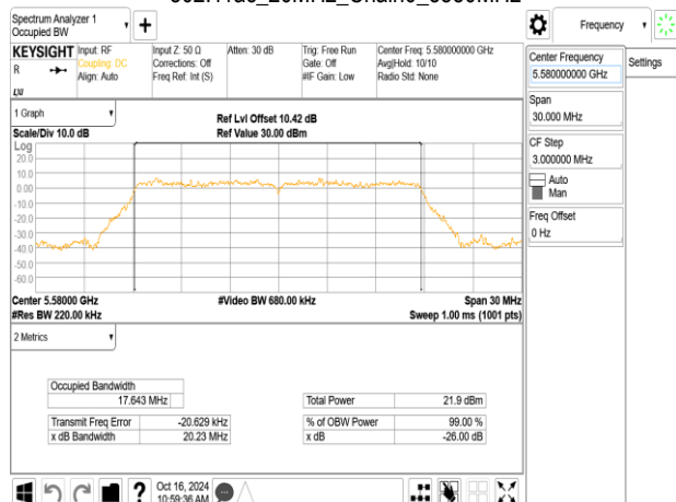
802.11ac_20MHz_Chain0_5580MHz
