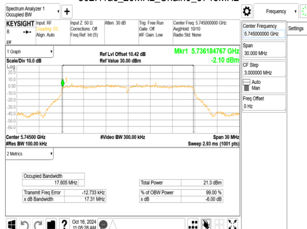
802.11ac_20MHz_Chain0_5745MHz
