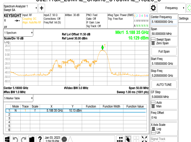
802.11ax_20MHz_Chain0_5180MHz_RU52_37
