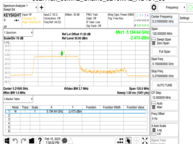
802.11ax_80MHz_Chain0_5210MHz_RU484_66
