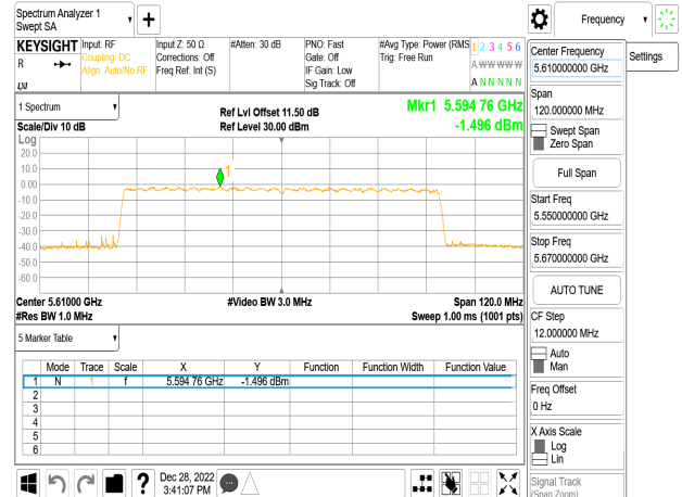
802.11ax_80MHz_Chain0_5610MHz_RU484_65
