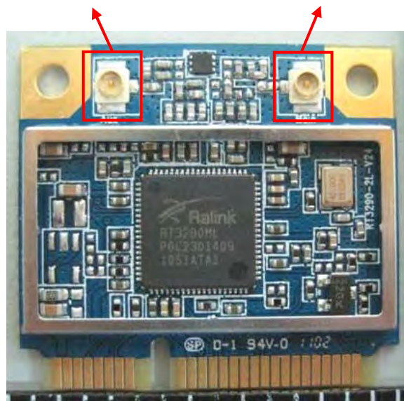
Connector 2: TX/RX (AUX port)
