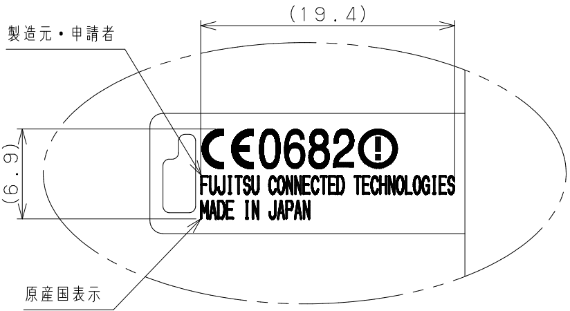
B 詳細図
