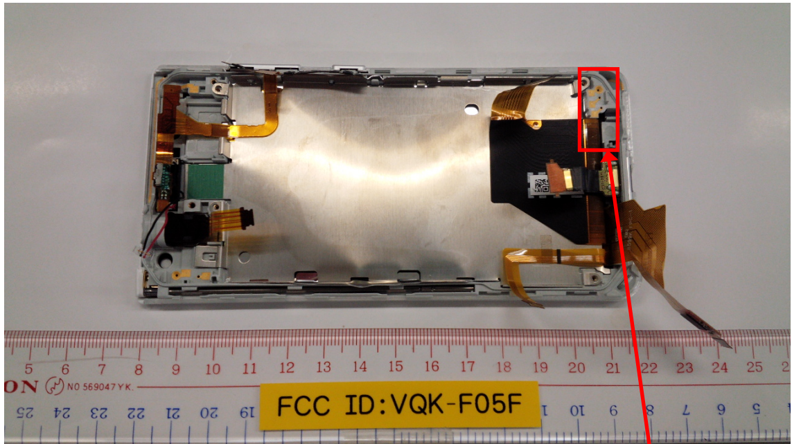
WWAN ANTENNA
