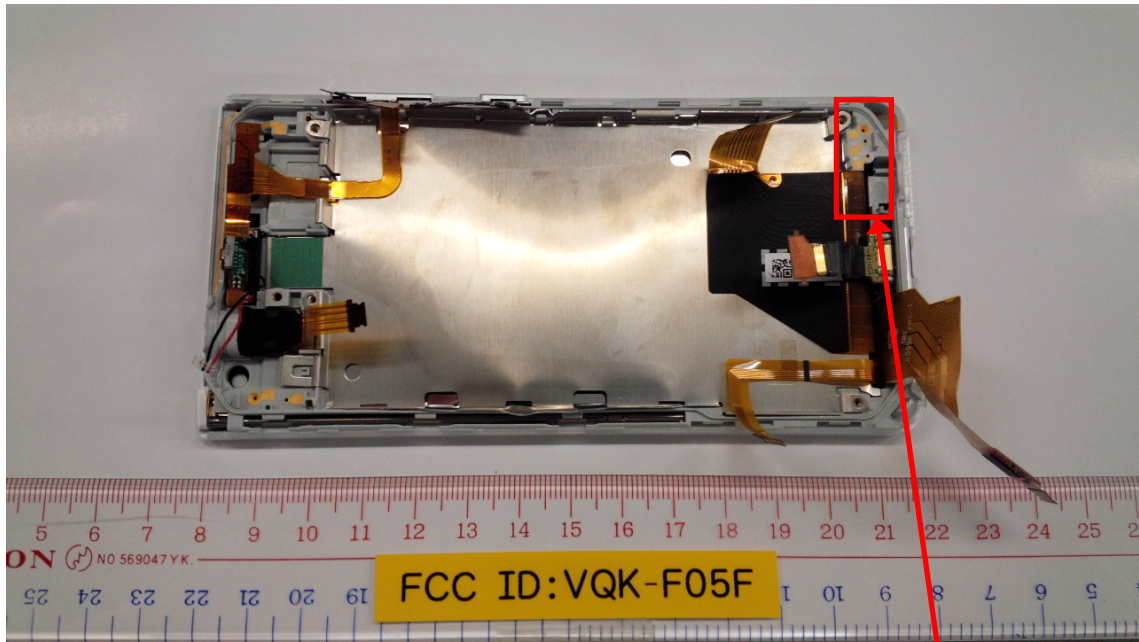
WWAN ANTENNA
