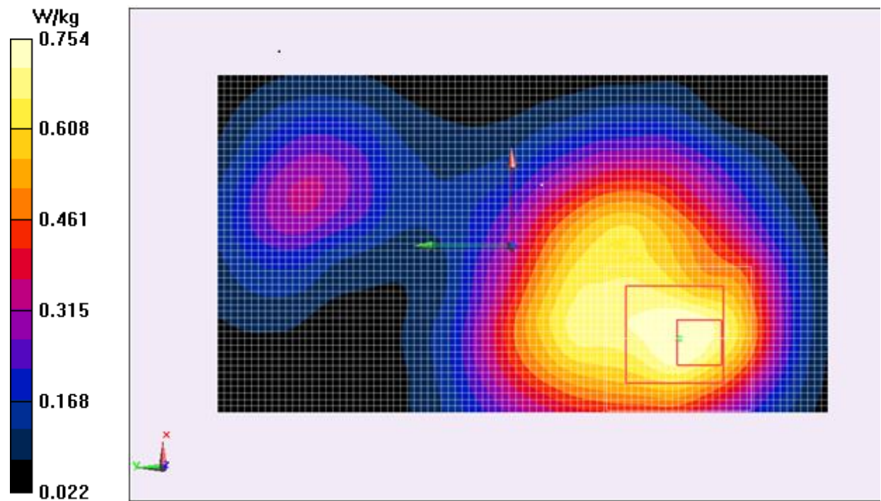
Fig.10 WCDMA1900 CH9262
