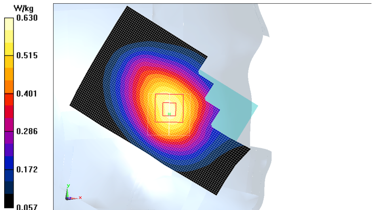
Fig.5 WCDMA 850
