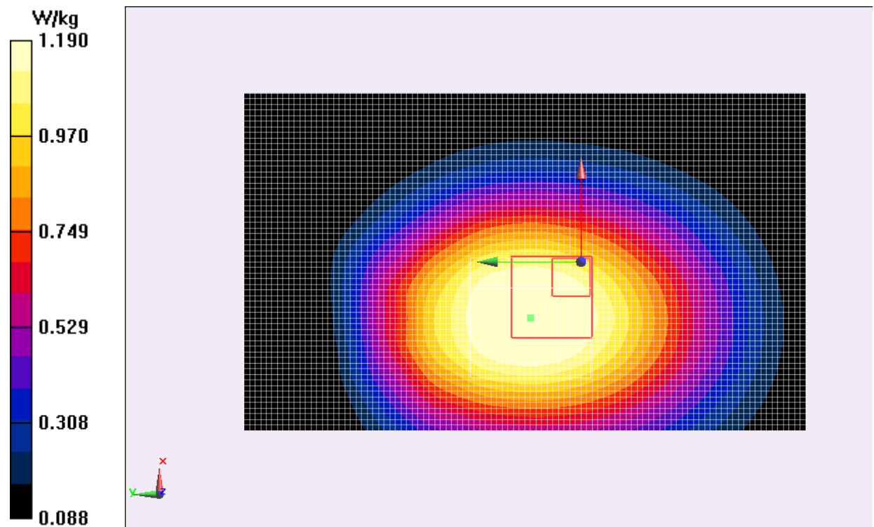
Fig.5 WCDMA 850 CH4183
