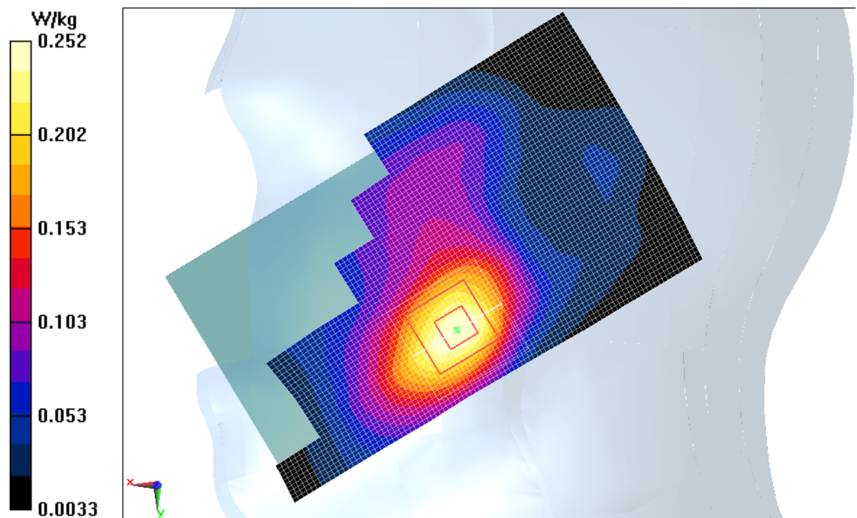
Fig.7 WCDMA1900 CH9538
