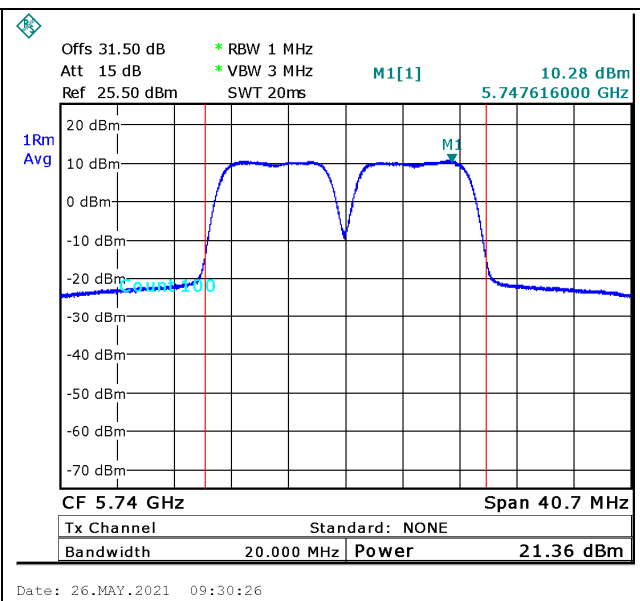
Figure 33. 5740.0MHz, 20MHz BW
