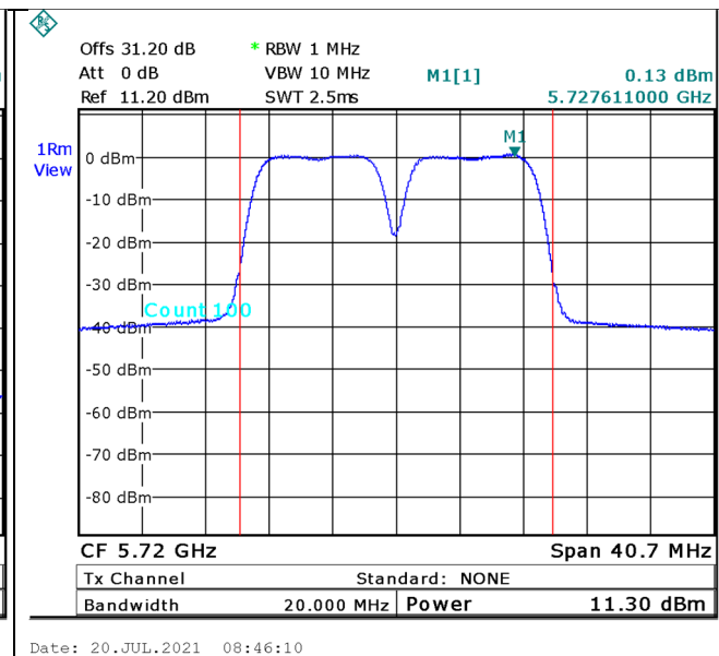
Figure 67. 5720.0MHz, 20MHz BW
