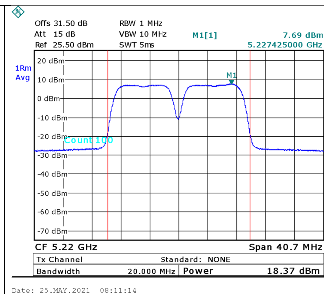
Figure 12. 5220.0MHz, 20MHz BW
