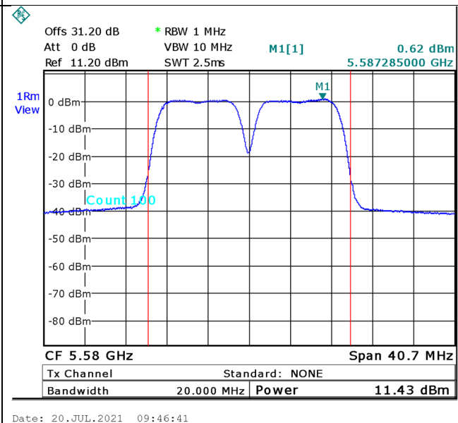
Figure 65. 5580.0MHz, 20MHz BW
