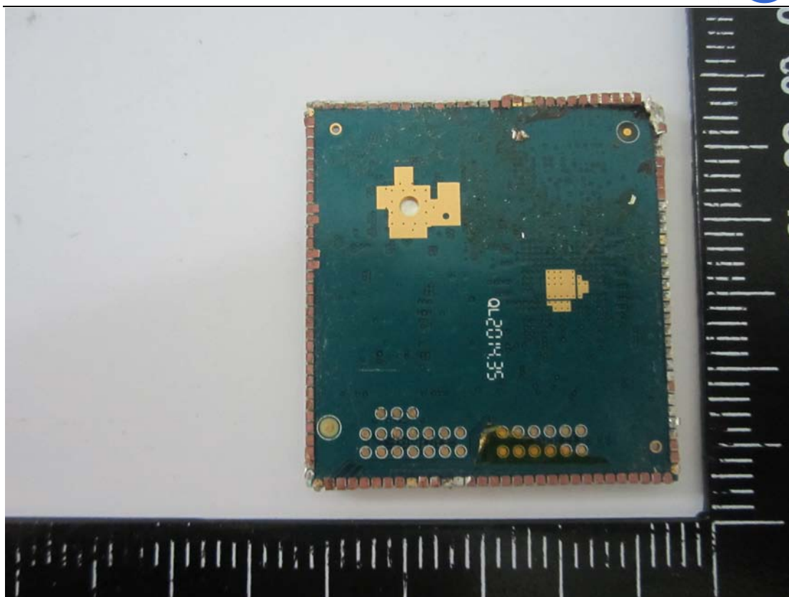
6. BT/WIFI antenna view
