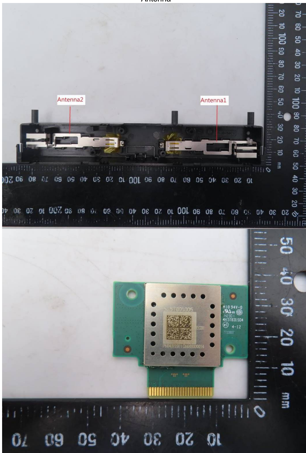
Antenna
