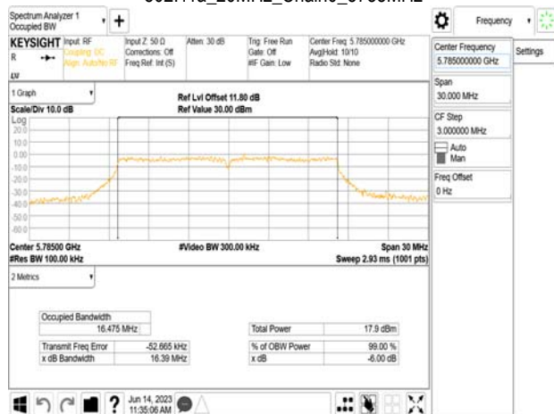
802.11a_20MHz_Chain0_5785MHz
