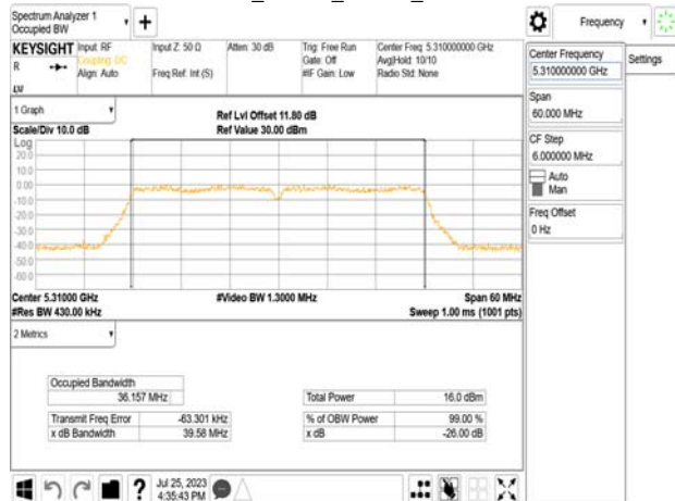
802.11n_40MHz_Chain1_5310MHz
