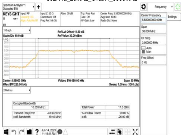
802.11a_20MHz_Chain1_5580MHz
