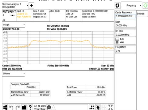
802.11a_20MHz_Chain0_5700MHz
