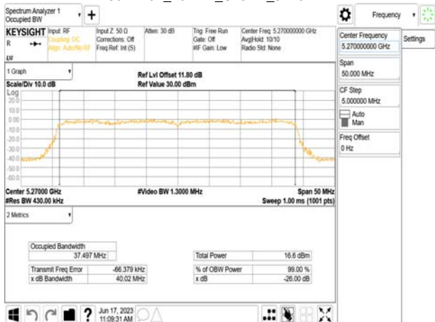
802.11ax_40MHz_Chain1_5270MHz
