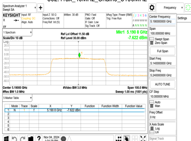
802.11ax_40MHz_Chain0_5190MHz_RU242_61
