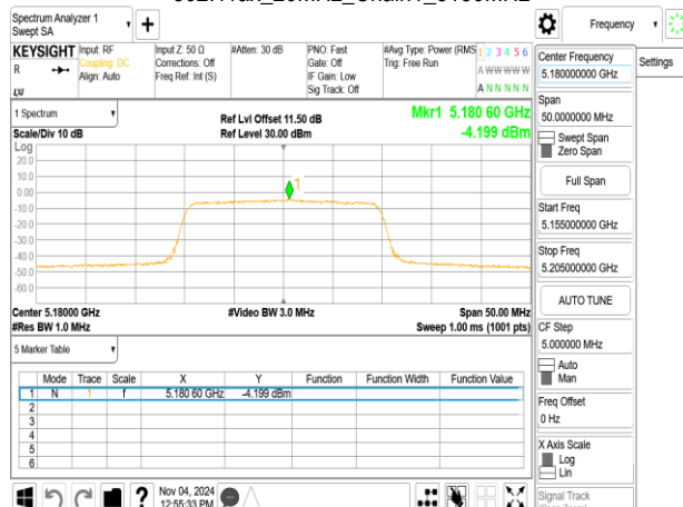
802.11ax_20MHz_Chain1_5180MHz_RU106_53
