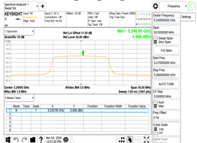
802.11ax_20MHz_Chain0_5240MHz
