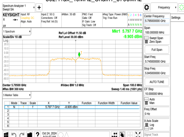
802.11ax_40MHz_Chain1_5795MHz_RU242_62
