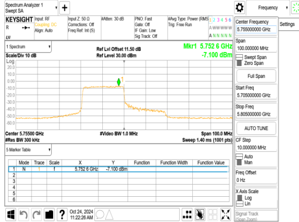
802.11ax_40MHz_Chain1_5755MHz_RU242_61
