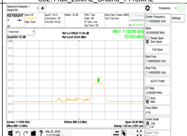
802.11ax_20MHz_Chain0_7115MHz_RU52_40
