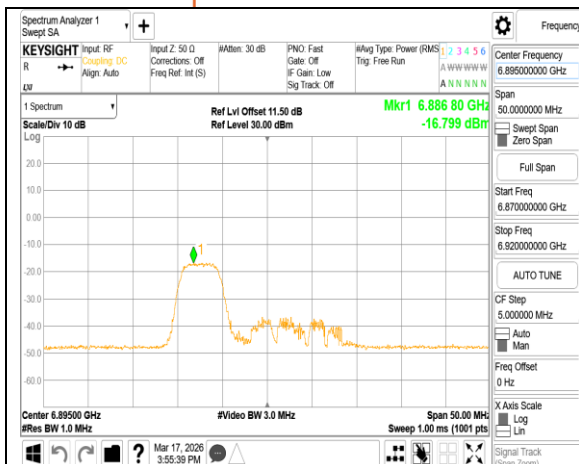
802.11ax_20MHz_Chain0_6895MHz_RU52_37
