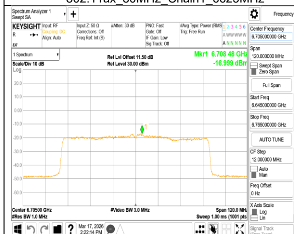
802.11ax_80MHz_Chain1_6705MHz
