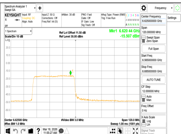
802.11ax_80MHz_Chain1_6625MHz_RU484_65
