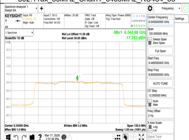
802.11ax_80MHz_Chain1_6545MHz
