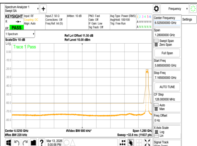
802.11ax 20MHz Chain1 7115MHz
