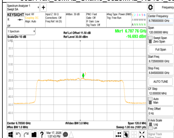
802.11ax 80MHz Chain0 6785MHz
