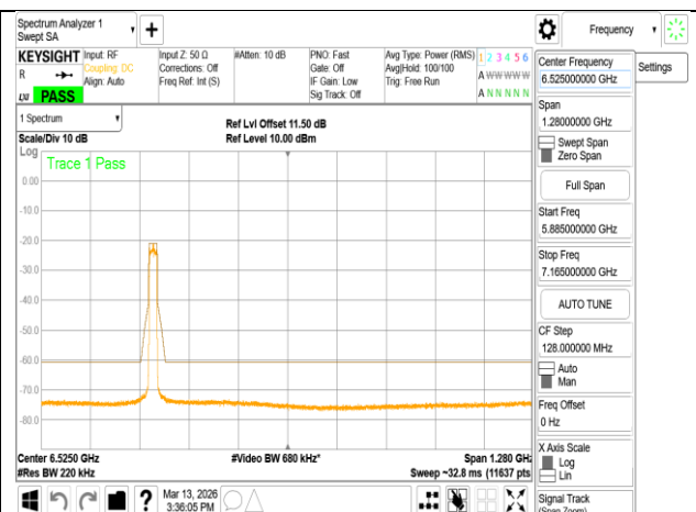
802.11ax_20MHz_Chain0_6175MHz
