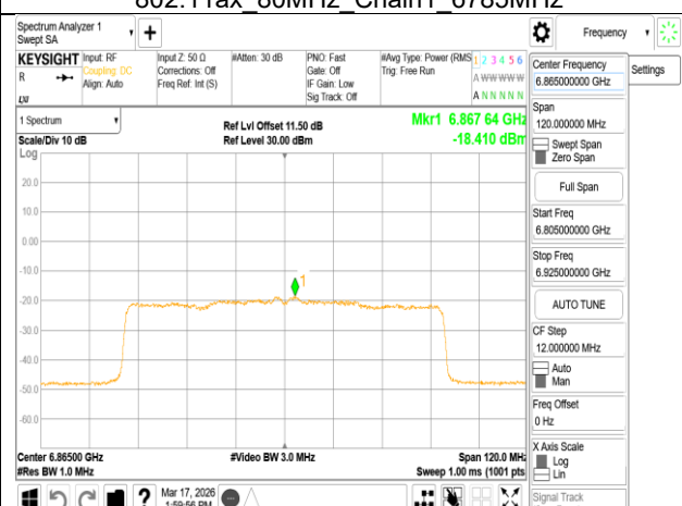
802.11ax_80MHz_Chain1_6865MHz
