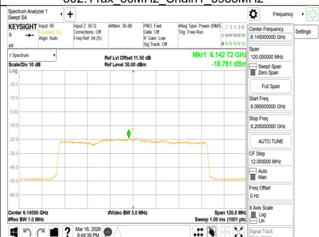
802.11ax 80MHz Chain1 6145MHz
