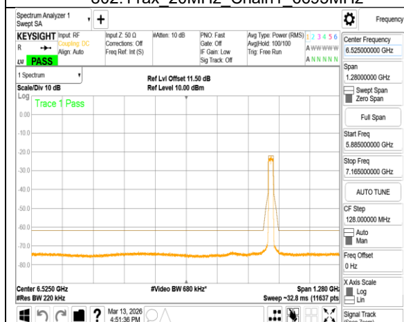
802.11ax 20MHz Chain1 6875MHz
