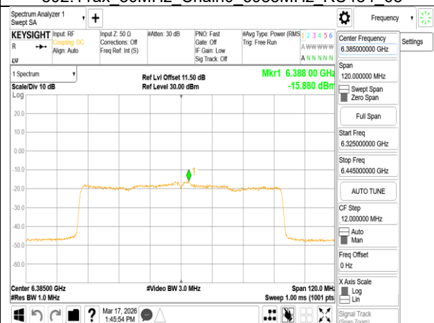
802.11ax_80MHz_Chain0_6385MHz
