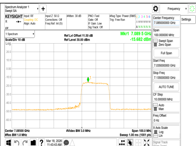
802.11ax_40MHz_Chain1_7085MHz_RU242_62
