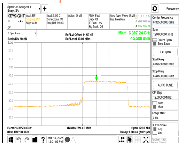
802.11ax 80MHz Chain0 6385MHz RU484 66
