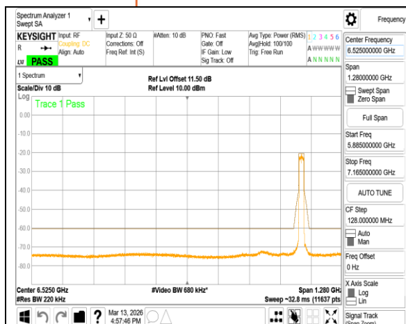
802.11ax 20MHz Chain1 6995MHz
