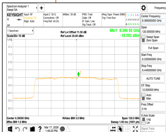
802.11ax_80MHz_Chain1_6385MHz
