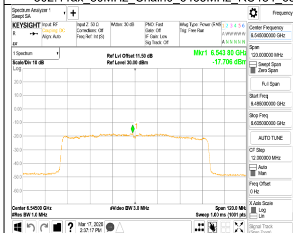
802.11ax 80MHz Chain0 6545MHz
