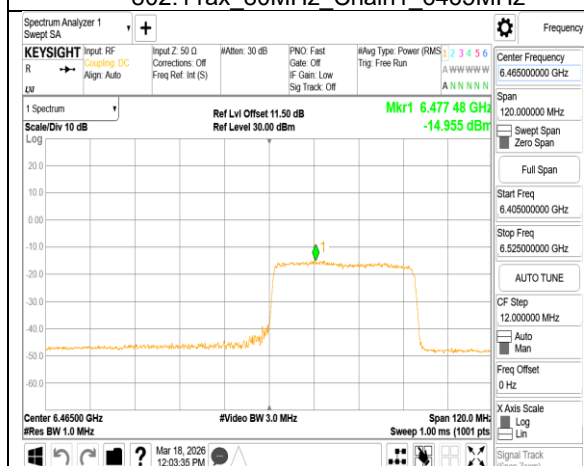
802.11ax_80MHz_Chain1_6465MHz_RU484_66
