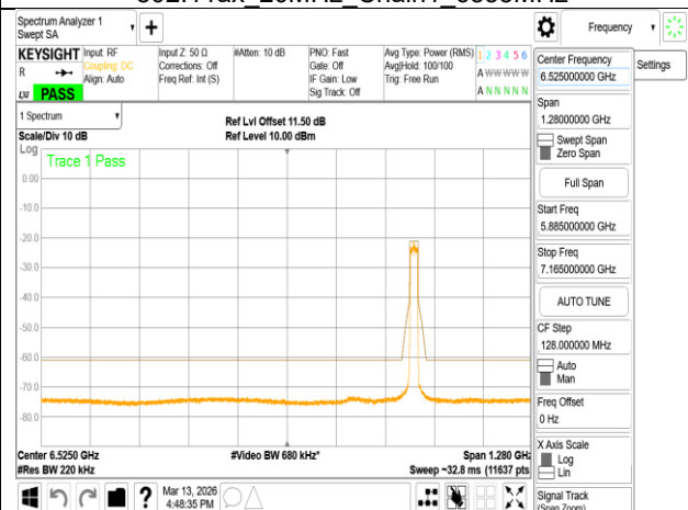
802.11ax 20MHz Chain1 6855MHz
