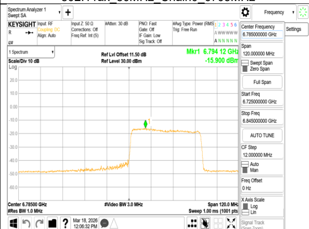
802.11ax 80MHz Chain0 6785MHz RU484 66
