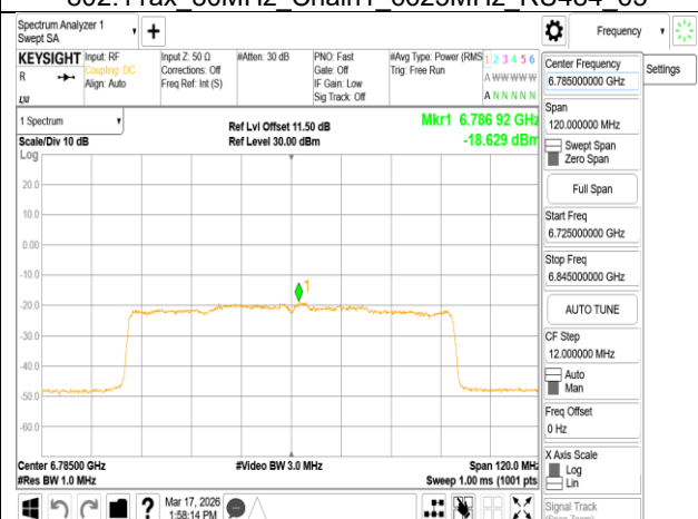
802.11ax_80MHz_Chain1_6785MHz
