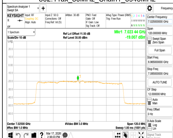
802.11ax 80MHz Chain1 7025MHz
