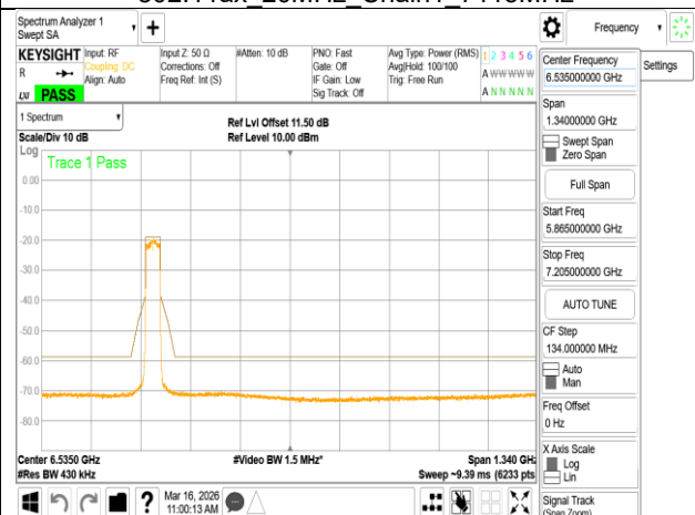
802.11ax 40MHz Chain0 6165MHz
