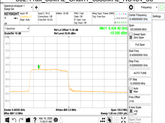
802.11ax_80MHz_Chain1_6465MHz_RU484_65
