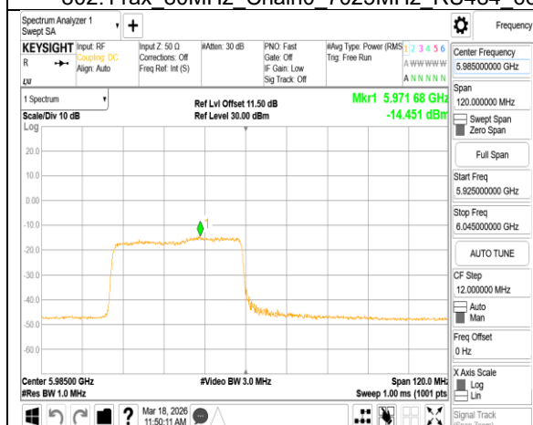
802.11ax 80MHz Chain1 5985MHz RU484 65
