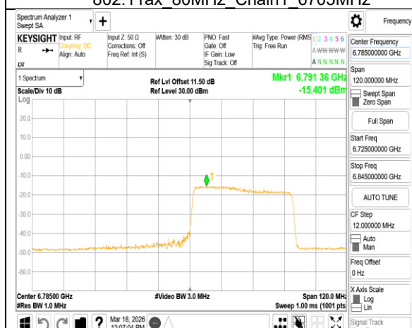
802.11ax_80MHz_Chain1_6785MHz_RU484_66
