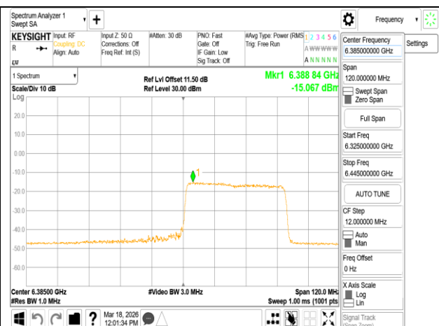
802.11ax_80MHz_Chain1_6385MHz_RU484_66
