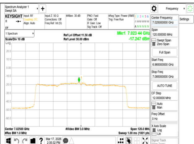
802.11ax 80MHz Chain0 7025MHz
