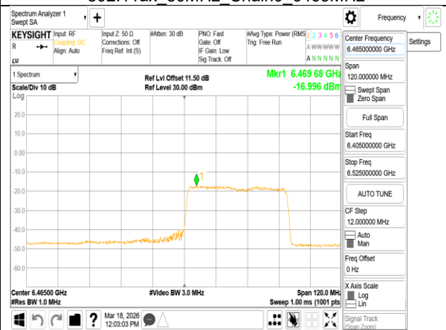
802.11ax 80MHz Chain0 6465MHz RU484 66
