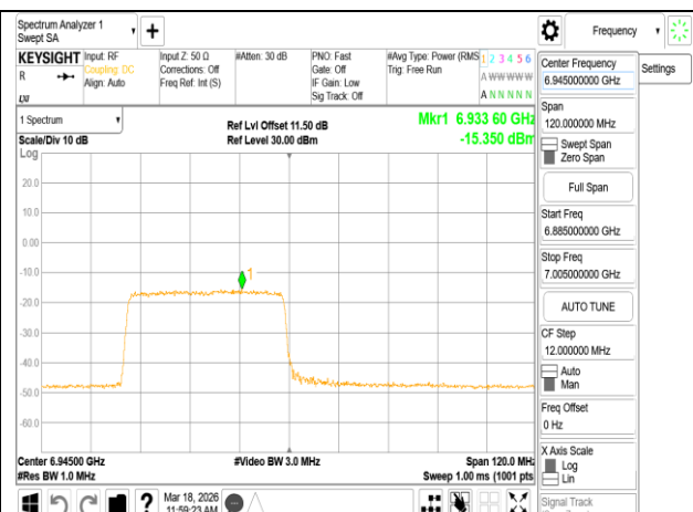
802.11ax 80MHz Chain1 6945MHz RU484 65
