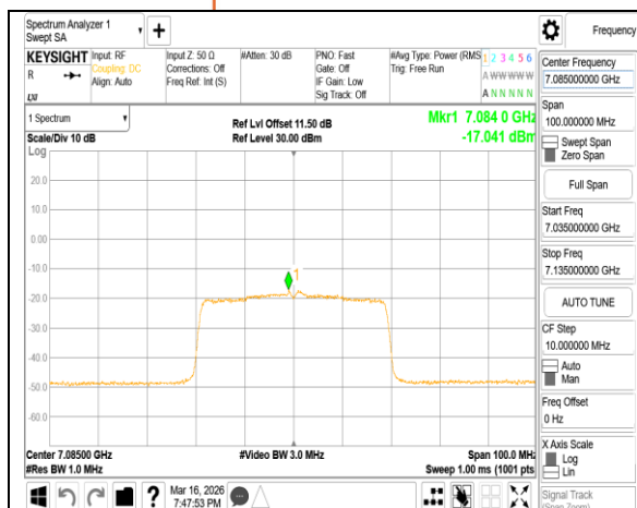
802.11ax_40MHz_Chain1_7085MHz
