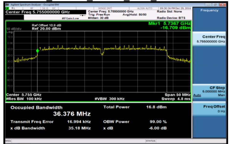
FCC 802.11n 40MHz Main 5755MHz
