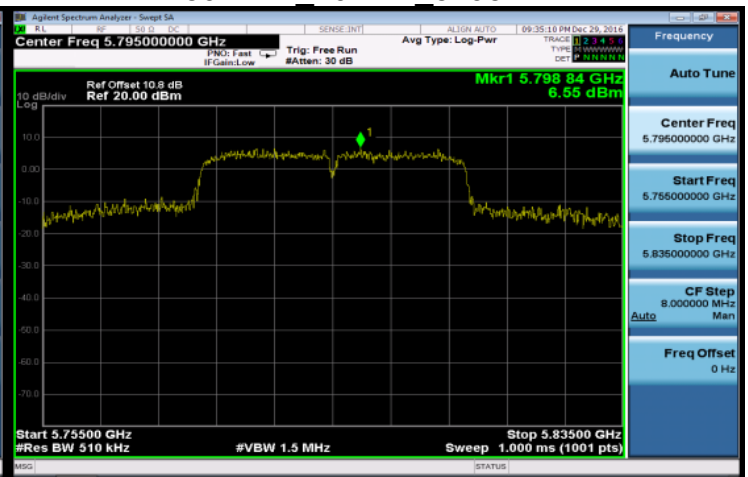
802.11n 40MHz 5795MHz
