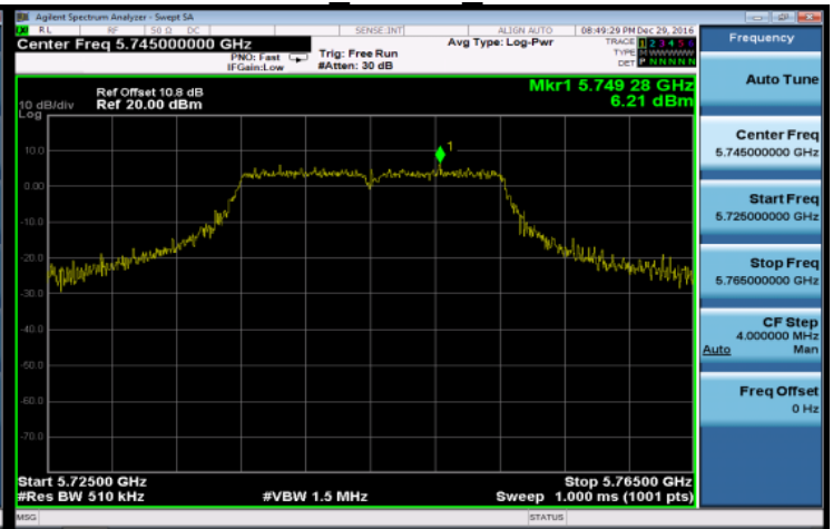
802.11a 20MHz 5745MHz
